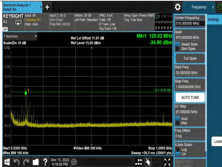
DH5-Ant1-2441-30~1000--10.60
