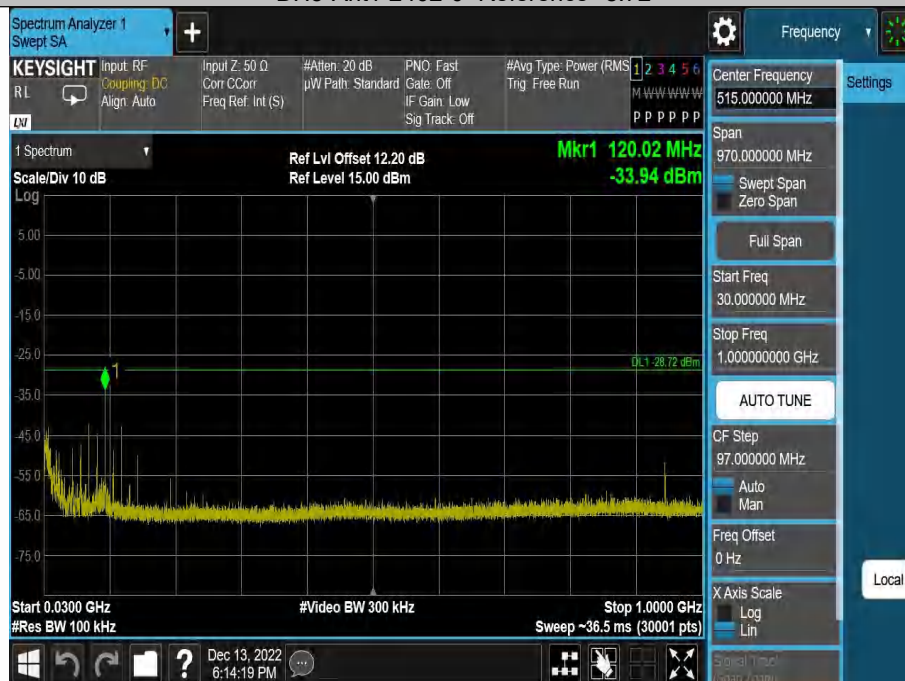
DH5-Ant1-2402-30~1000--8.72
