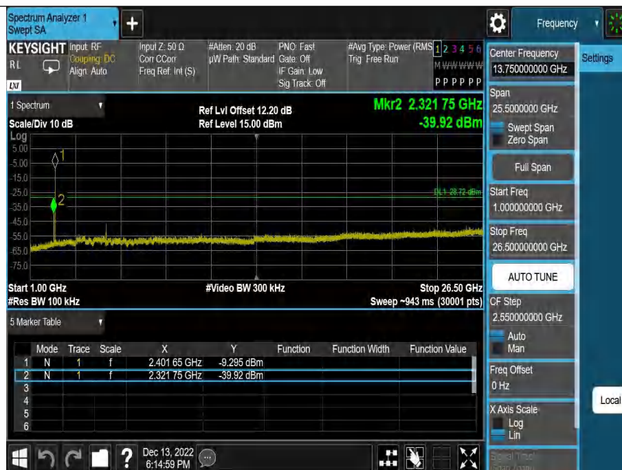
DH5-Ant1-2402-1000~26500~-8.72
