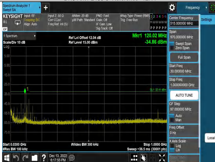
DH5-Ant1-2480-30~1000--12.41
