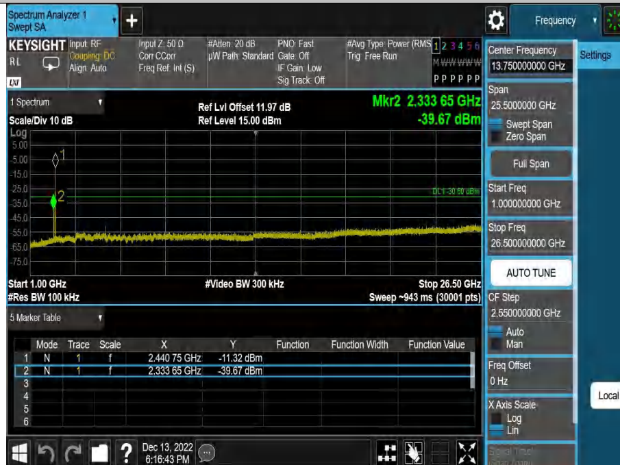
DH5-Ant1-2441-1000~26500--10.60
