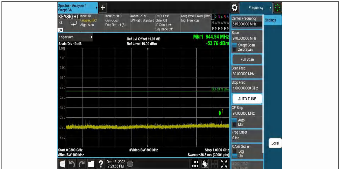
DH5-Ant1-2441-30~1000--8.73
