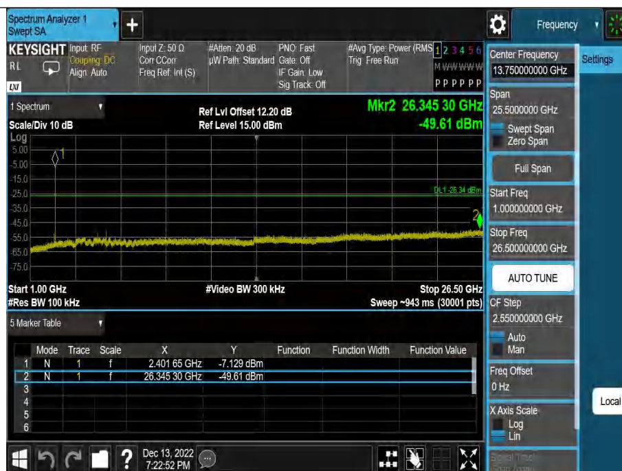
DH5-Ant1-2402-1000~26500~-6.34
