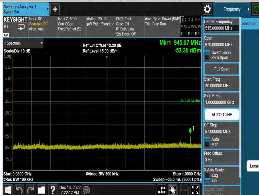
DH5-Ant1-2402-30~1000--6.34
