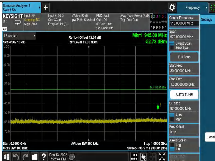
DH5-Ant1-2480-30~1000--10.57
