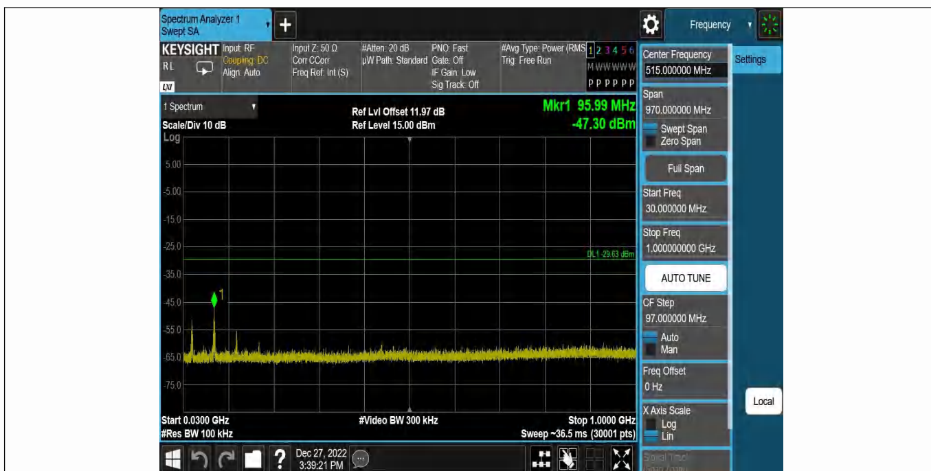
DH5-Ant1-2441-30~1000--9.63
