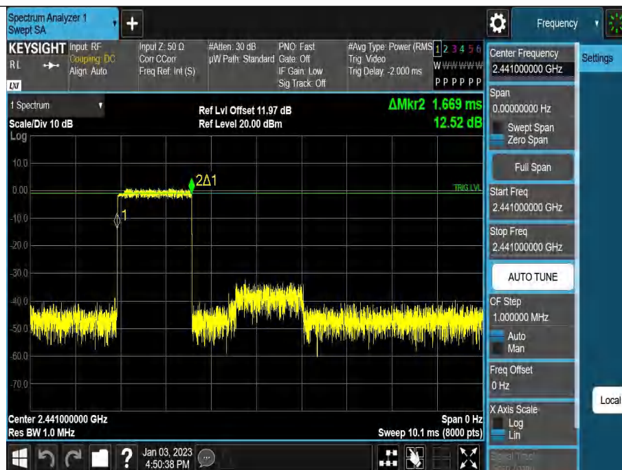
2DH3-Ant1-Hop-1.669-160
