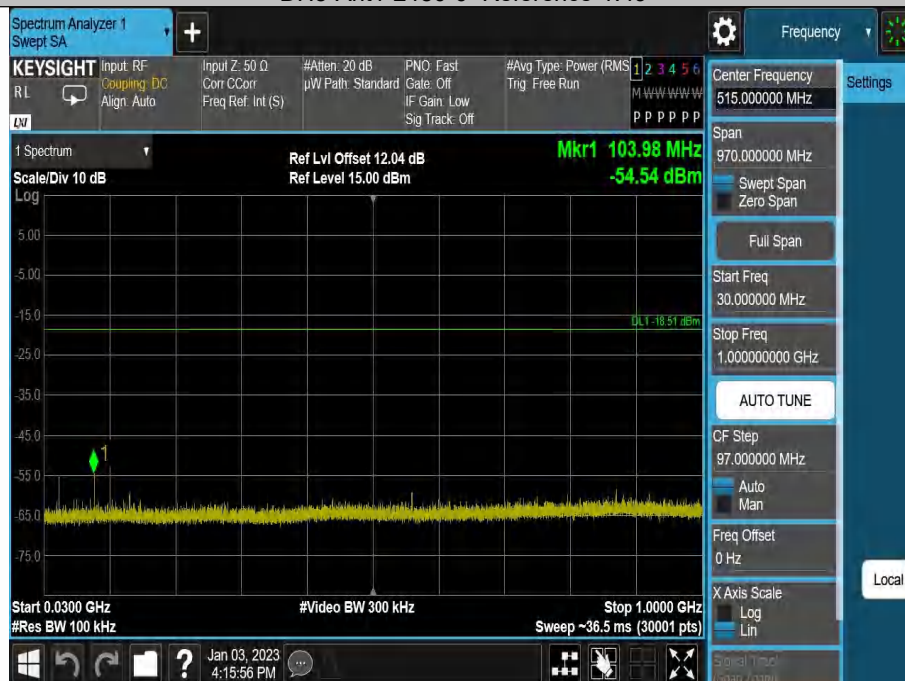
DH5-Ant1-2480-30~1000-1.49
