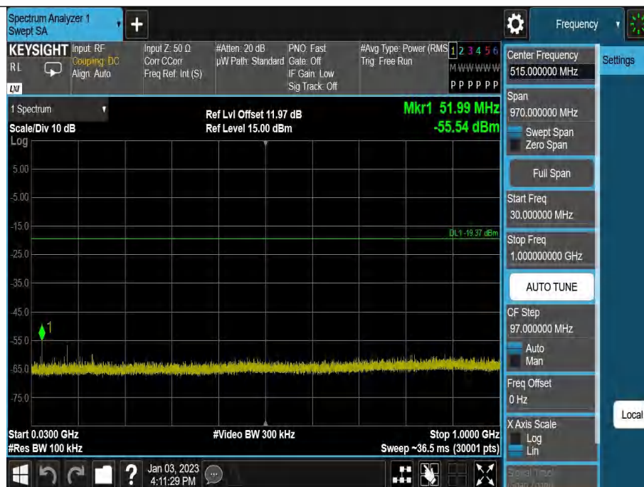
DH5-Ant1-2441-30~1000-0.63
