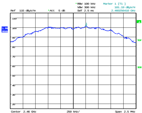
2460 MHz
