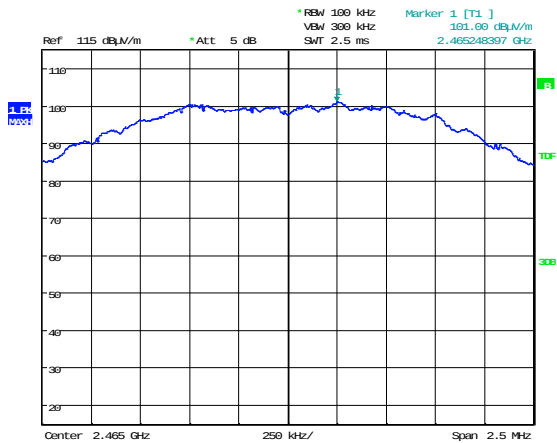
2465 MHz
