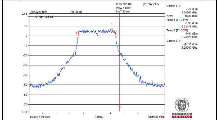
802.11a_Chain 3 / CH48
