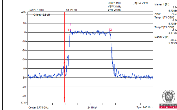
802.11ax (HE80)_Chain 3 / CH155
