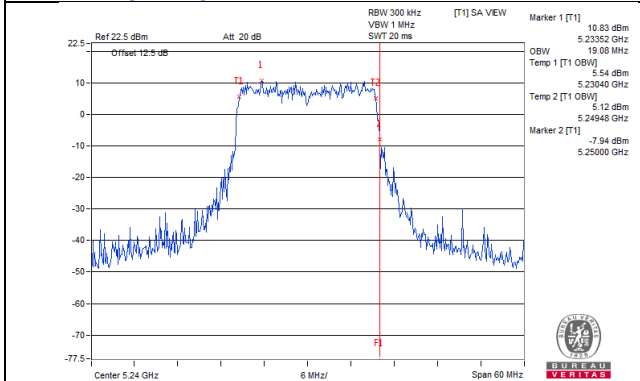
802.11ax (HE20)_Chain 4 / CH48
