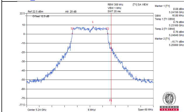
802.11a_Chain 6 / CH48
