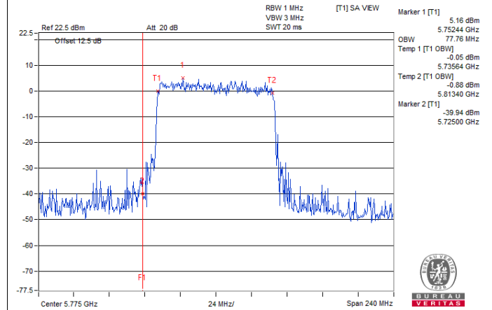
802.11ax (HE80+80) / Chain 3 : CH155
