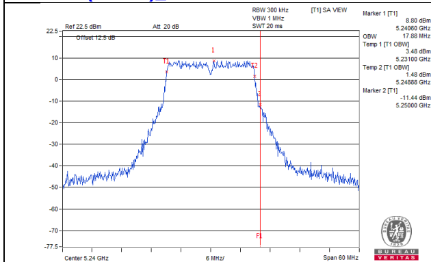
802.11ac (VHT20)_Chain 4 / CH48
