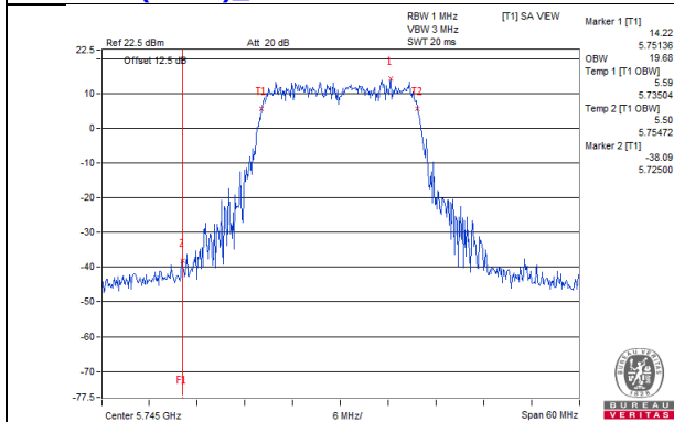
802.11ax (HE20)_Chain 6 / CH149
