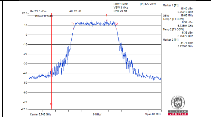
802.11ax (HE20)_Chain 3 / CH149
