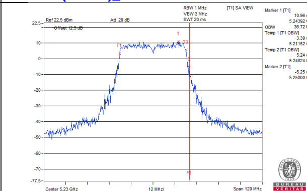
802.11ac (VHT40)_Chain 7 / CH46
