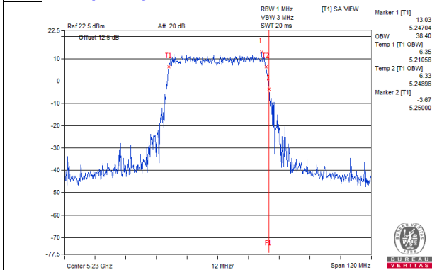
802.11ax (HE40)_Chain 4 / CH46
