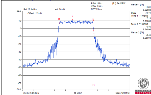
802.11ax (HE40)_Chain 6 / CH46
