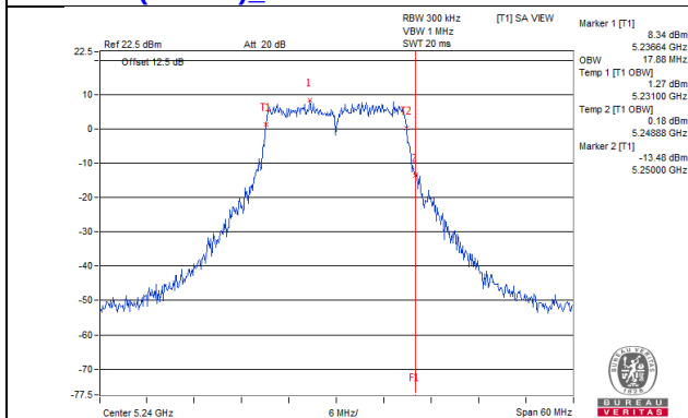
802.11ac (VHT20)_Chain 6 / CH48
