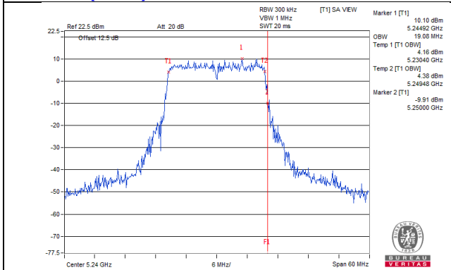
802.11ax (HE20)_Chain 6 / CH48
