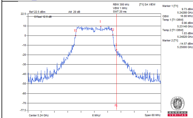
802.11a_Chain 4 / CH48
