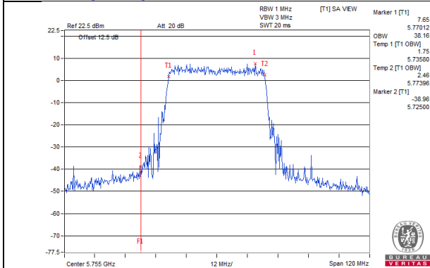
802.11ax (HE40)_Chain 4 / CH151
