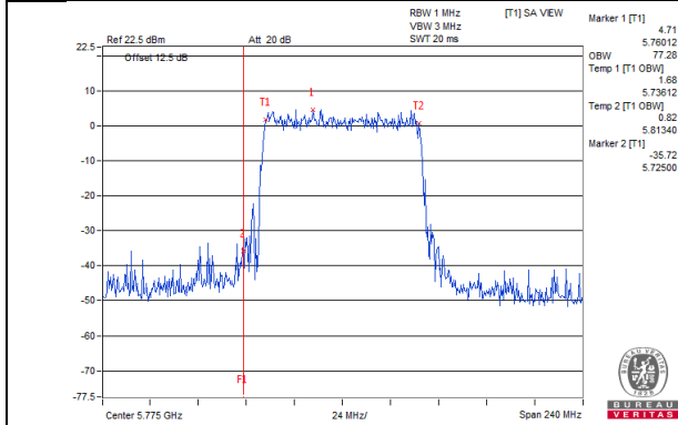
802.11ax (HE80)_Chain 4 / CH155
