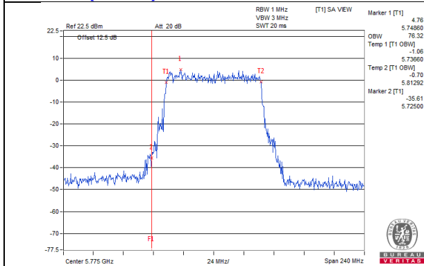
802.11ac (VHT80)_Chain 4 / CH155
