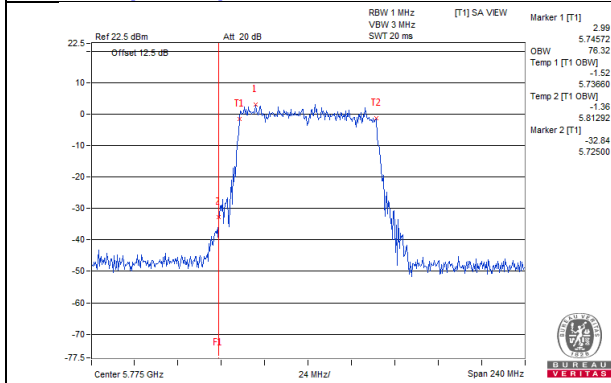
802.11ac (VHT80)_Chain 2 / CH155
