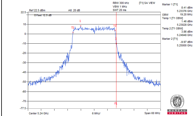
802.11ax (HE20)_Chain 2 / CH48
