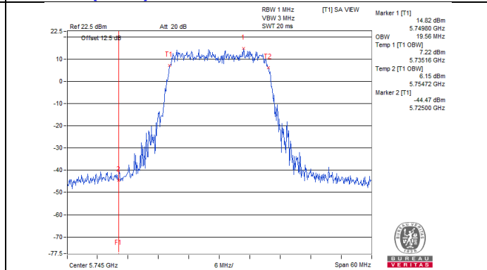
802.11ax (HE20)_Chain 5 / CH149
