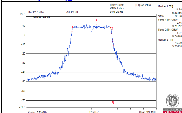
802.11ac (VHT40)_Chain 6 / CH46
