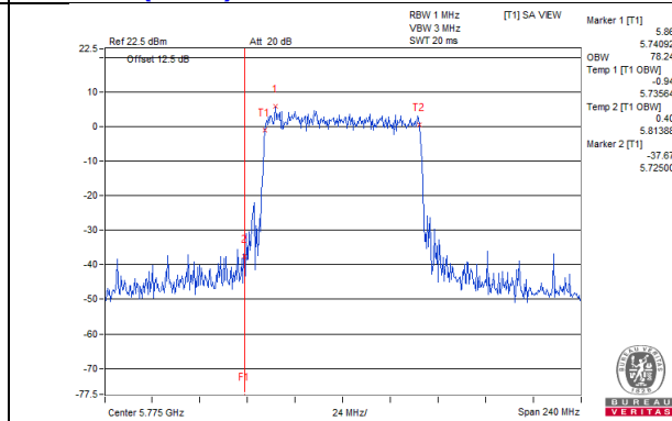
802.11ax (HE80)_Chain 7 / CH155
