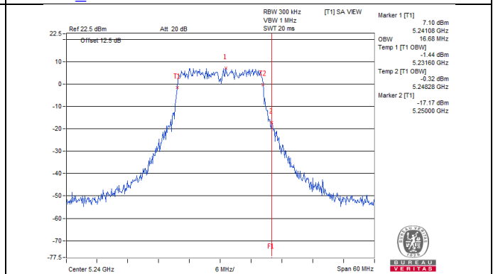
802.11a_Chain 7 / CH48
