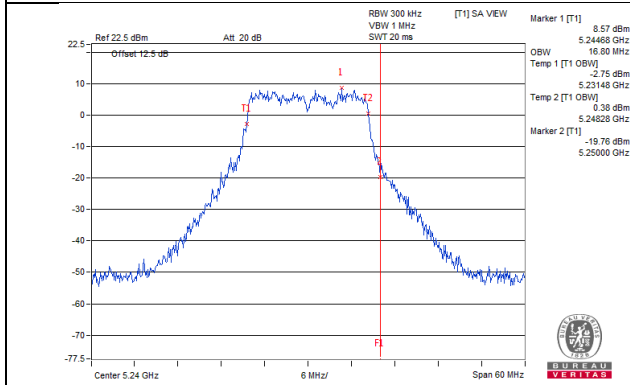
802.11a_Chain 2 / CH48
