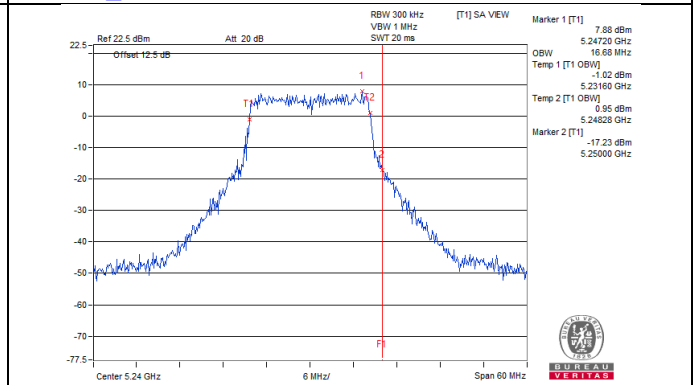
802.11a_Chain 5 / CH48
