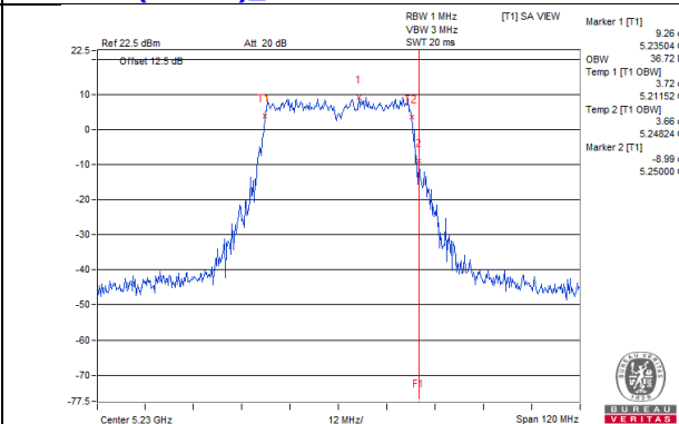
802.11ac (VHT40)_Chain 5 / CH46
