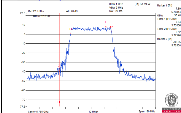
802.11ax (HE40)_Chain 6 / CH151
