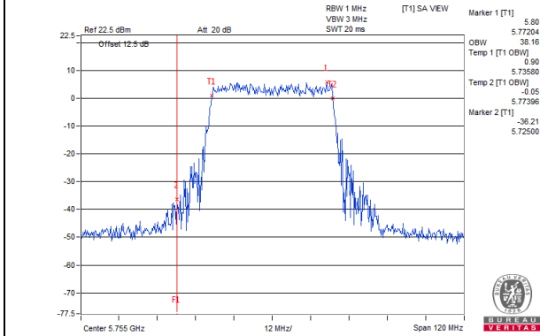
802.11ax (HE40)_Chain 2 / CH151
