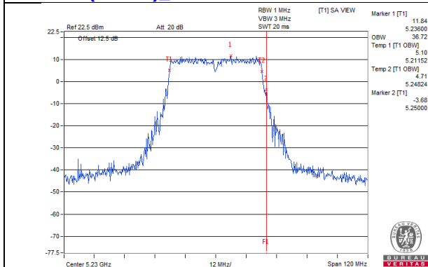
802.11ac (VHT40)_Chain 4 / CH46
