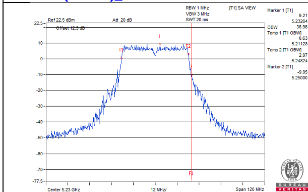
802.11ac (VHT40)_Chain 2 / CH46
