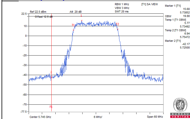
802.11ax (HE20)_Chain 4 / CH149
