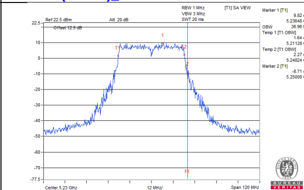
802.11ac (VHT40)_Chain 3 / CH46
