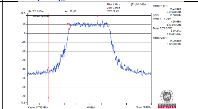
802.11ax (HE20)_Chain 7 / CH149
