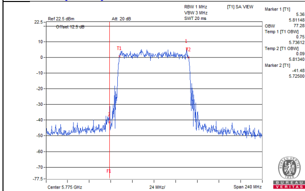
802.11ax (HE80)_Chain 6 / CH155
