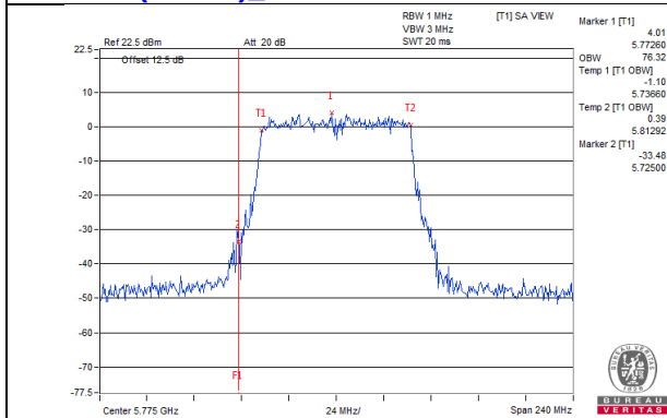
802.11ac (VHT80)_Chain 6 / CH155
