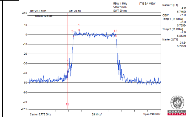
802.11ax (HE80)_Chain 5 / CH155
