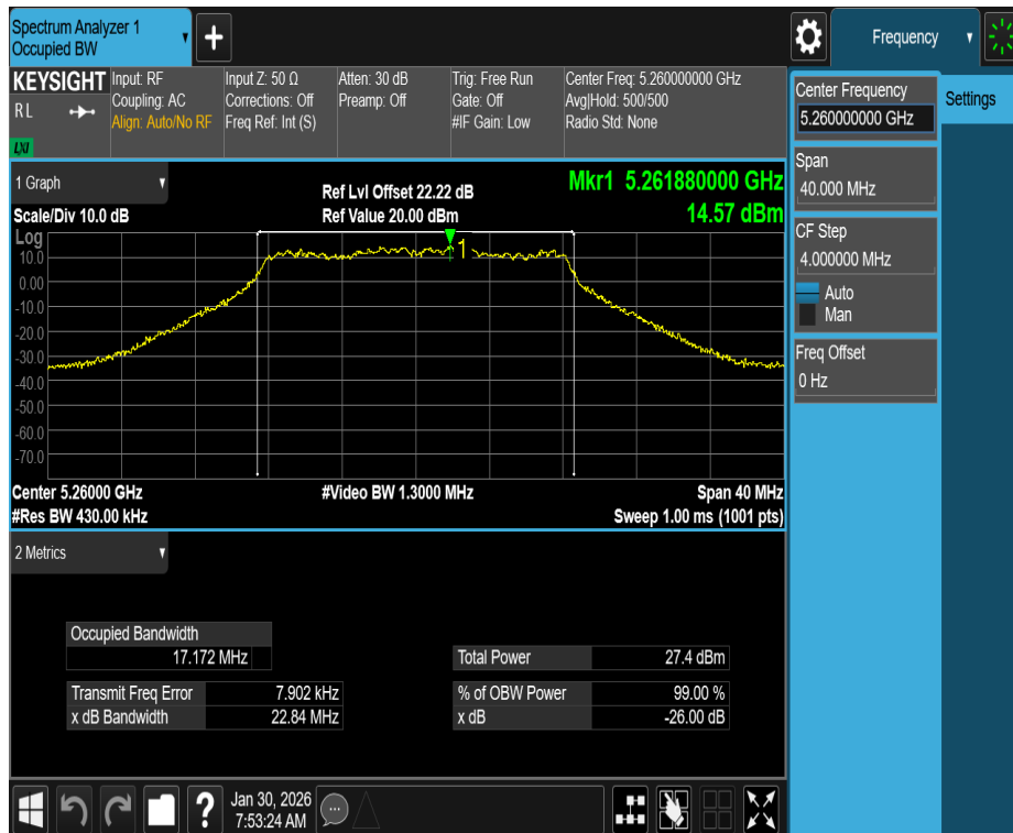
11A-CDD_Ant1_5260
