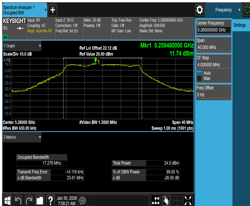
11A-CDD_Ant1_5260
