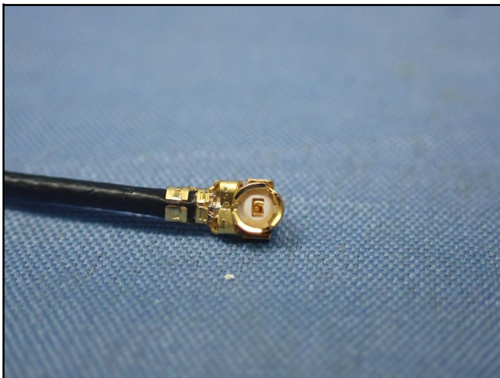
Ant: 5G2
