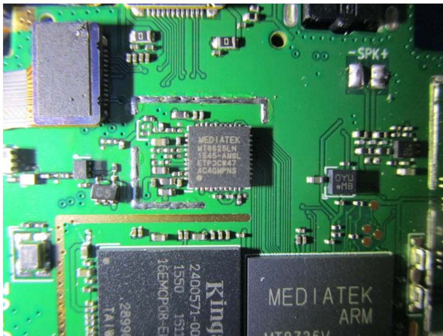
EUT –Wife&BT&GPS&FM View
