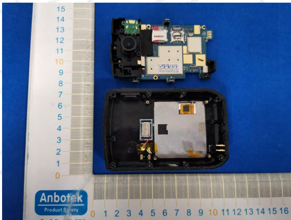
BT&WIFI ANT
