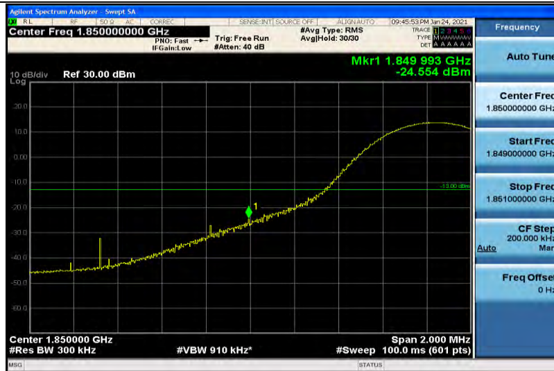
Band2-15MHz-QPSK-18675-1RB#74
