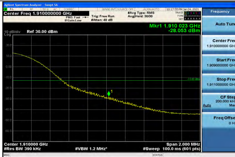
Band2-20MHz-QPSK-19100-1RB#0
