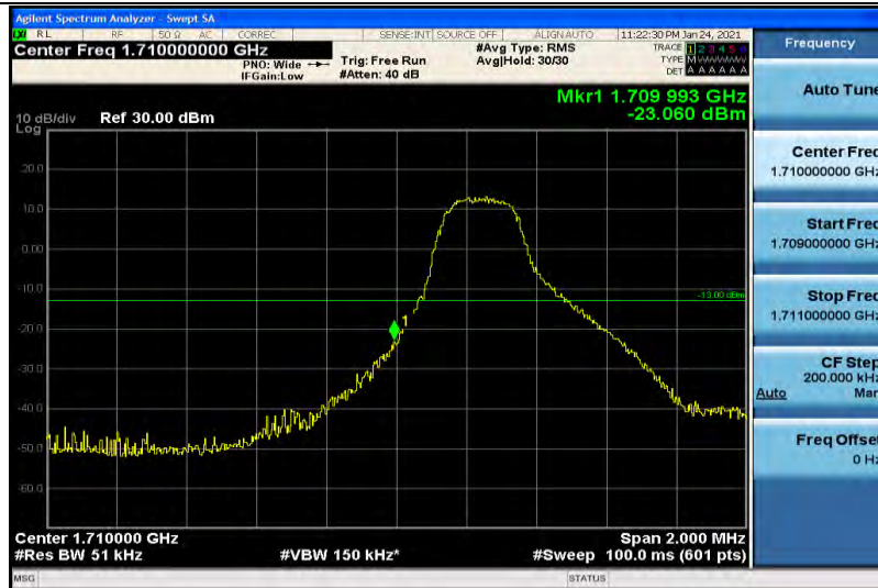
Band4-3MHz-QPSK-19965-1RB#14
