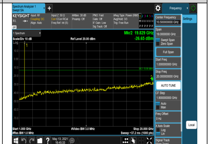
Band66-20MHz-QPSK-132072-1RB#0-Range2:1000~2
