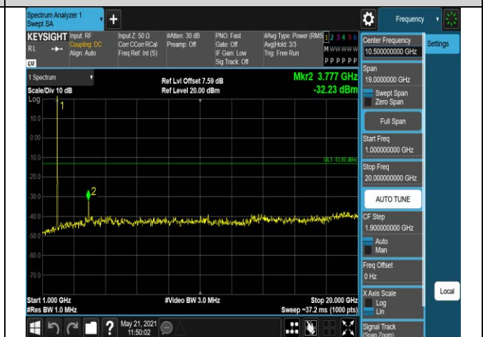
Band4-1.4MHz-QPSK-19957-1RB#0-Range2:1000~20
