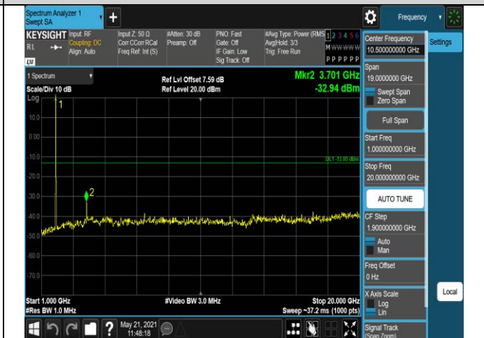
Band2-20MHz-16QAM-18900-1RB#0-Range2:1000~20
