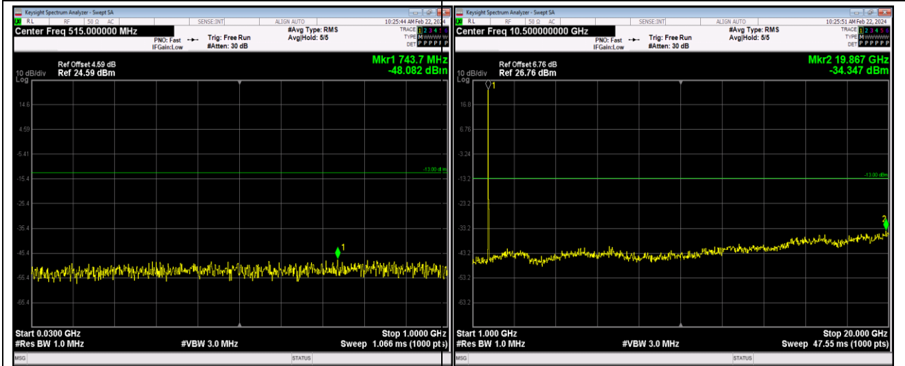
Band4-20MHz-QPSK-20300-1RB#0-Range1:30~1 000MHz
