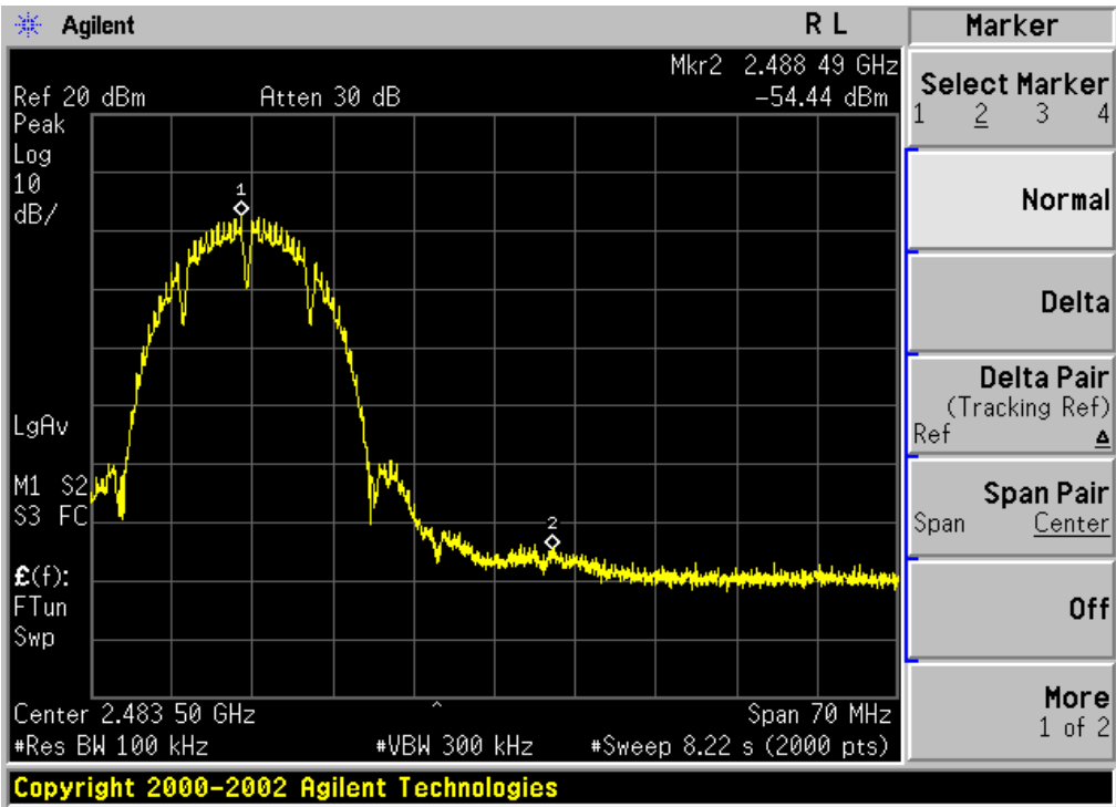
802.11b-CH11
