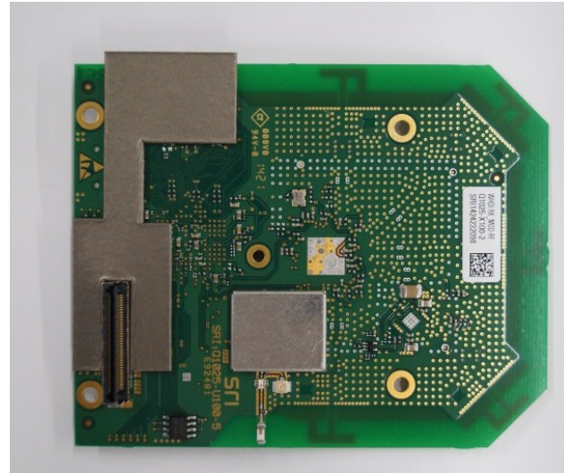
Q1025 – bottom side open shielding
