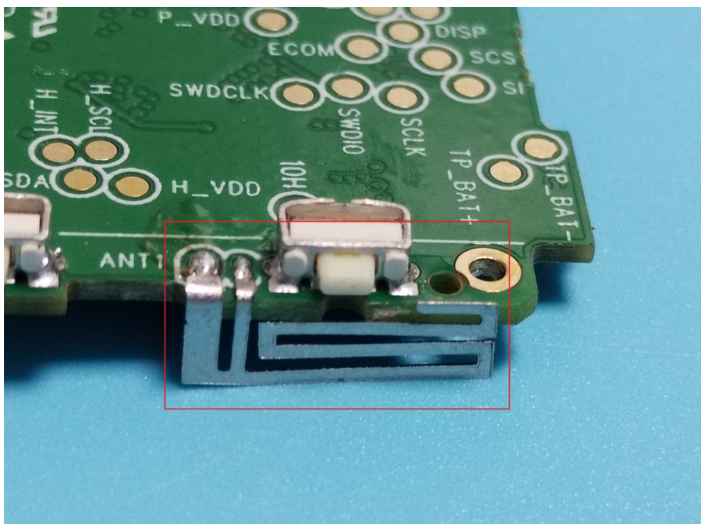
BLE ANT
