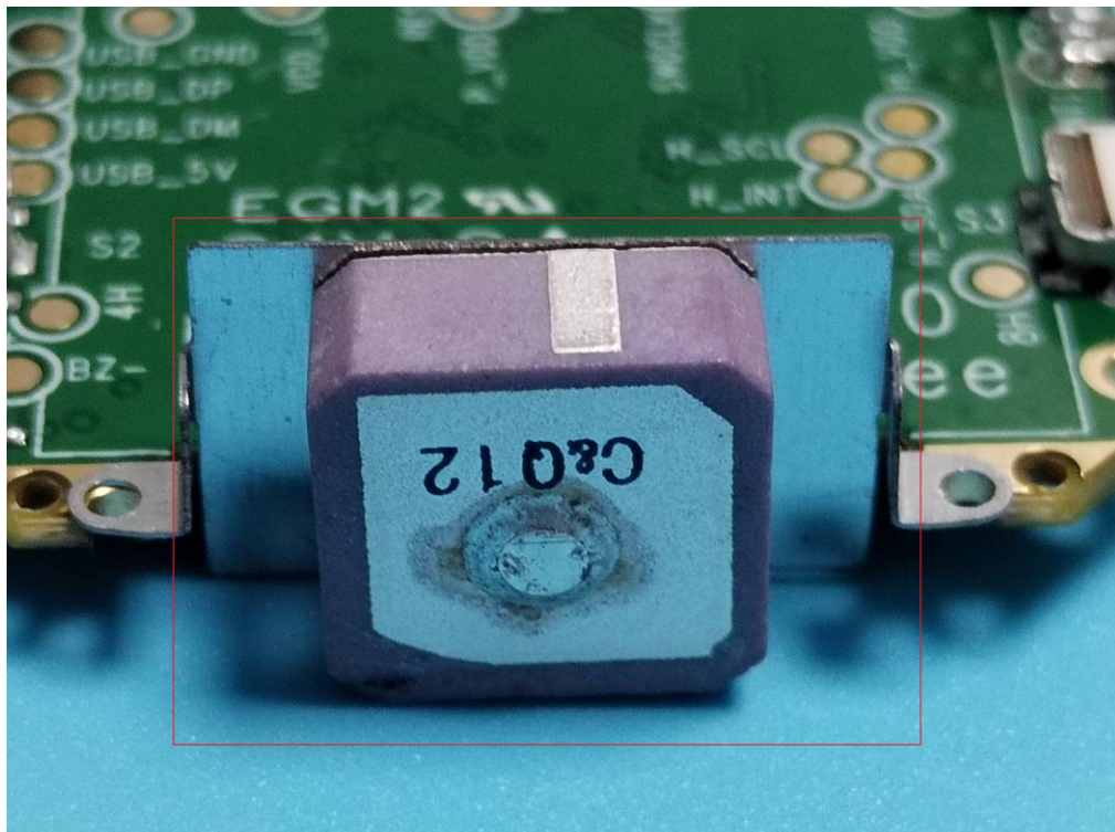
BLE ANT
