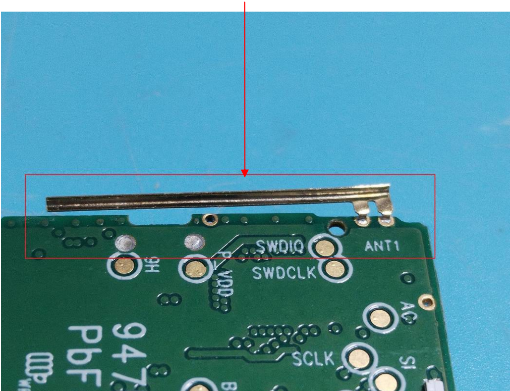
BLE ANT
