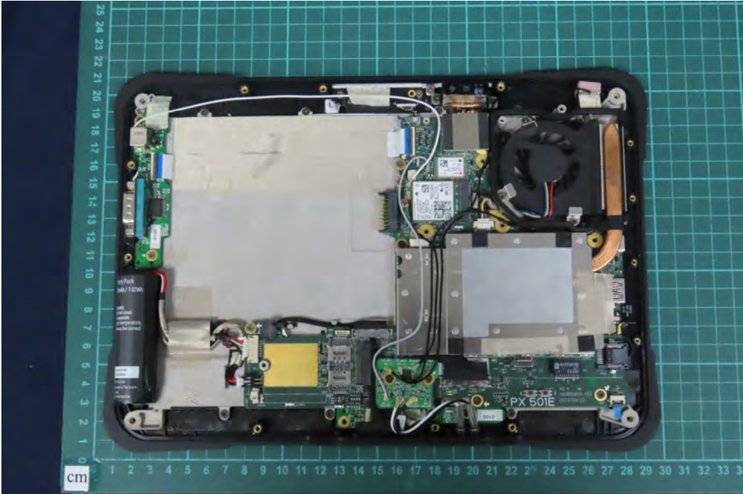
(13) EUT Photo
