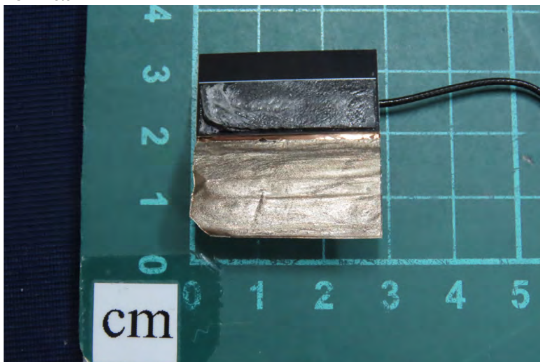
(40) EUT Photo
