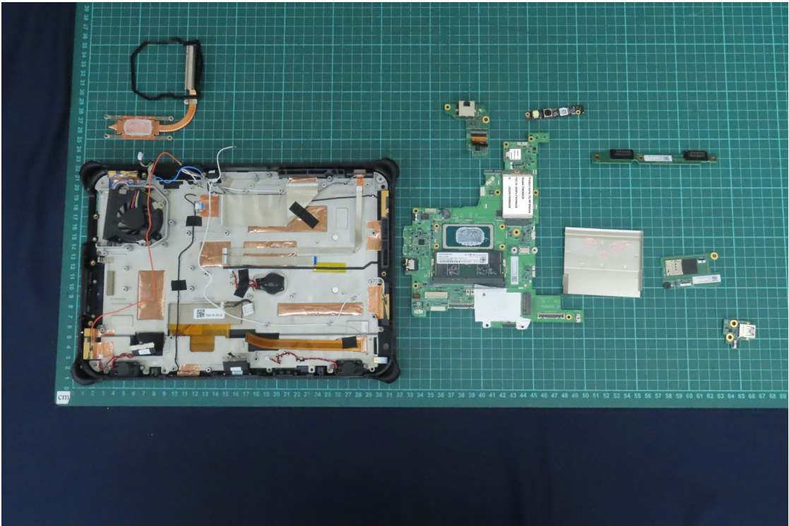
(21) EUT Photo
