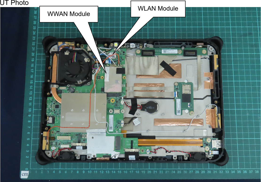
(20) EUT Photo
