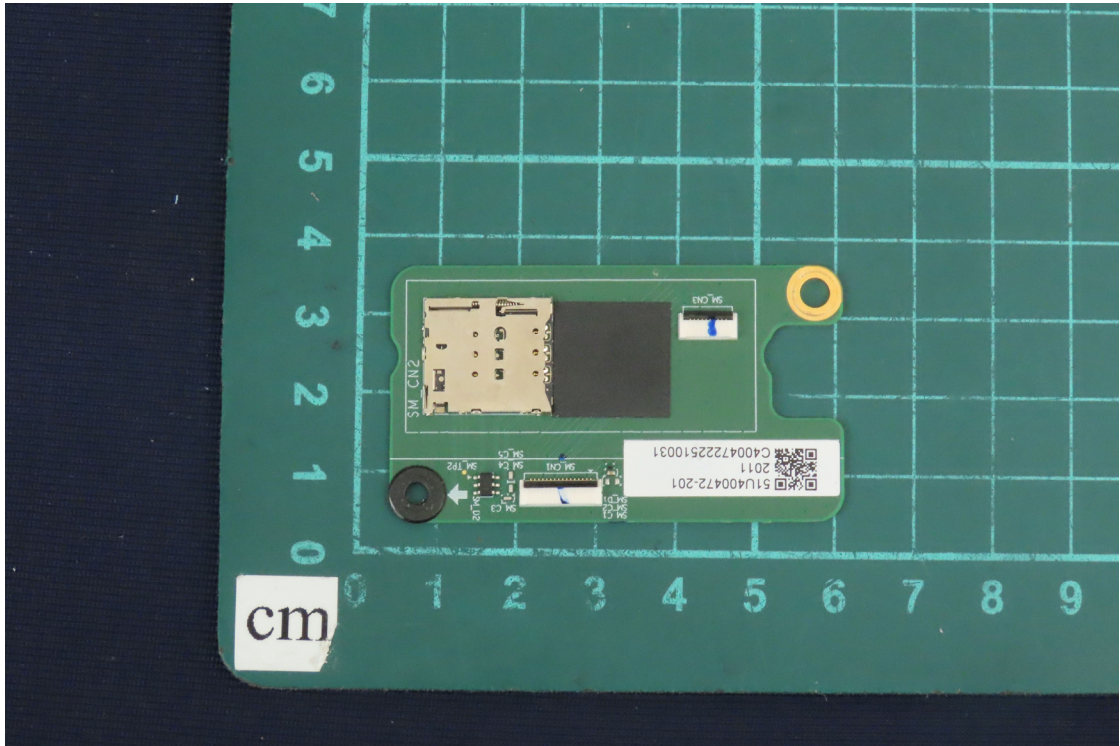
(24) EUT Photo
