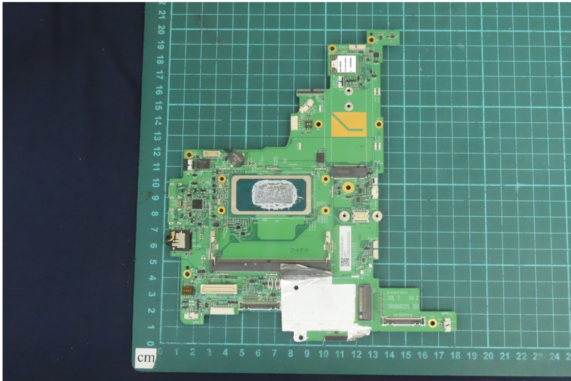
(37) EUT Photo
