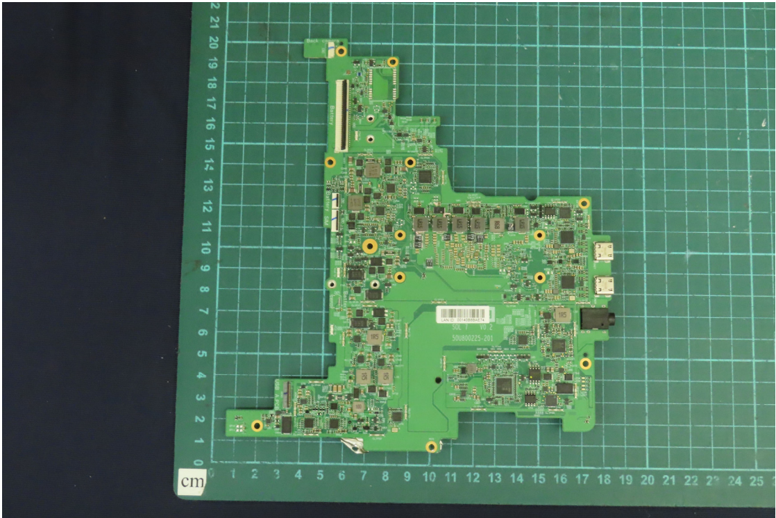
(44) EUT Photo
