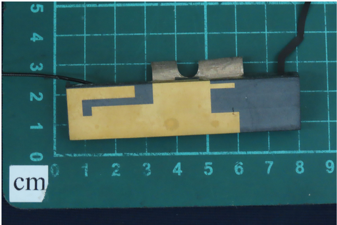
(57) EUT Photo
