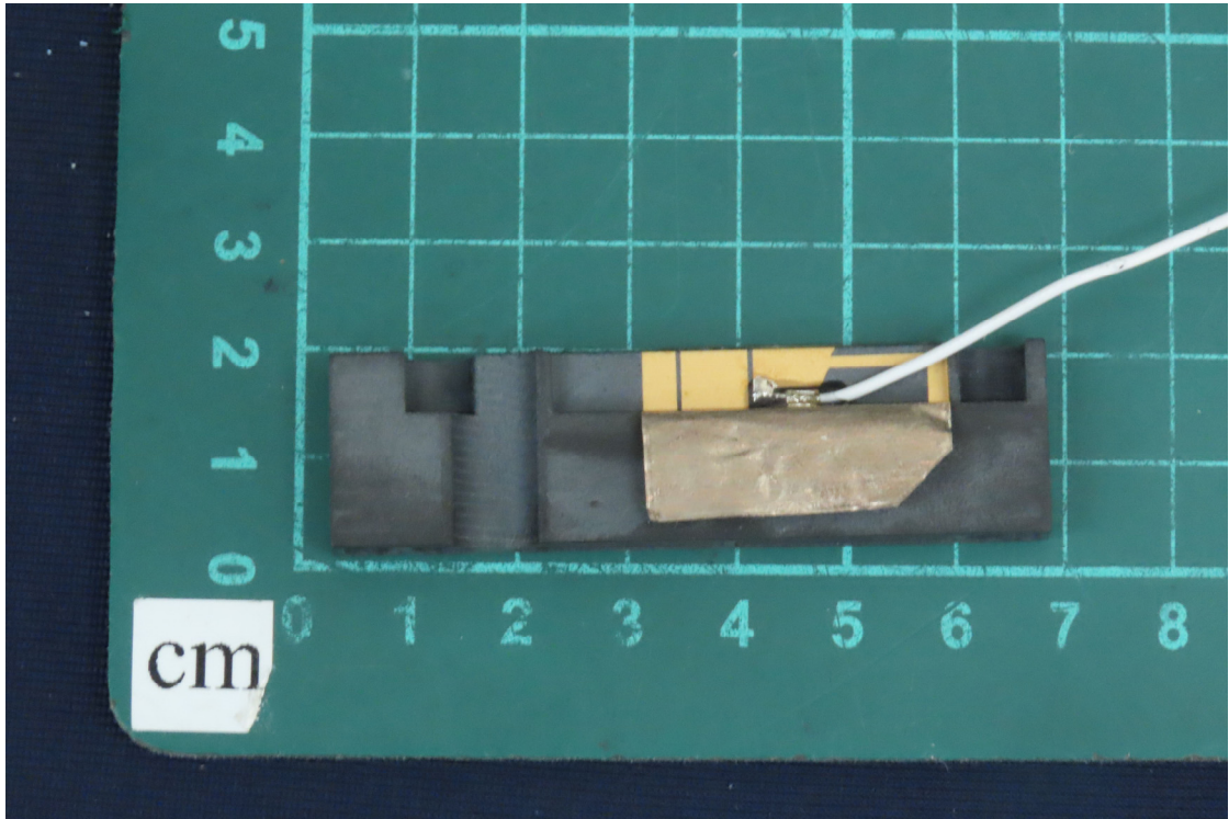
(59) EUT Photo
