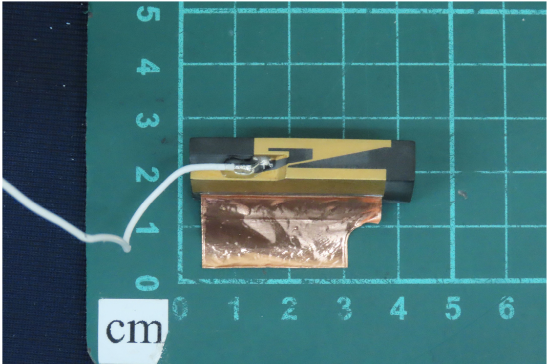
(52) EUT Photo
