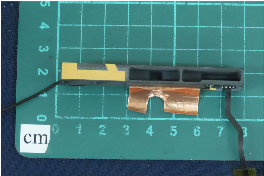
(56) EUT Photo
