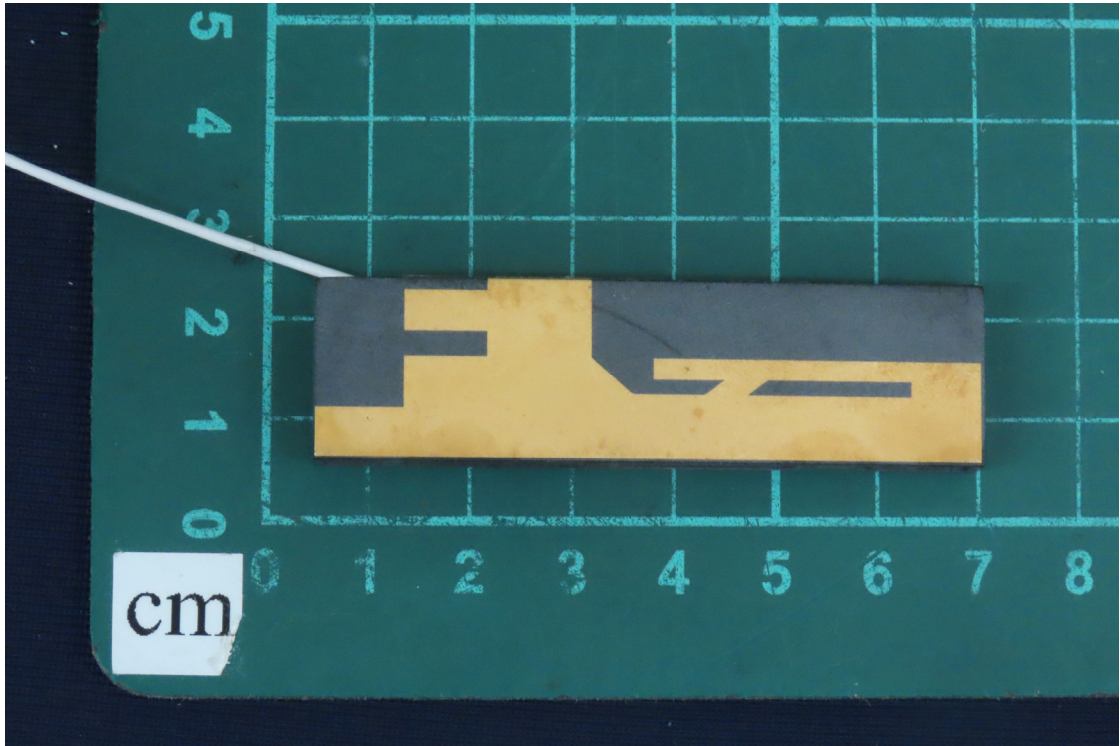
(58) EUT Photo
