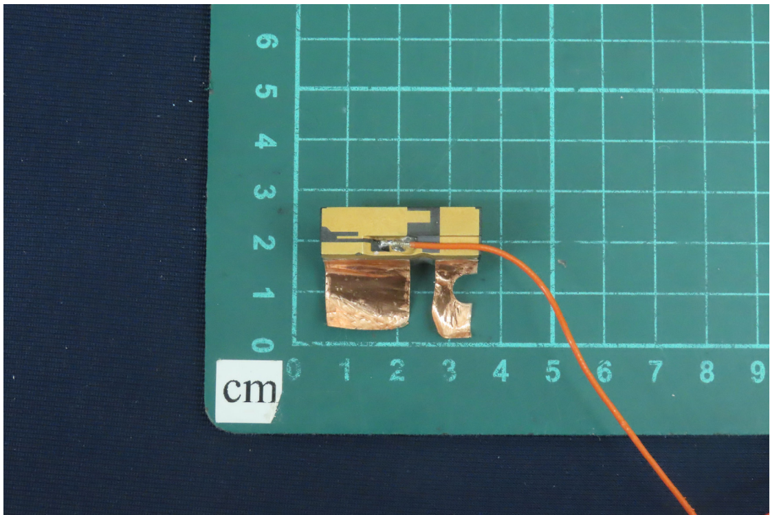
(62) EUT Photo
