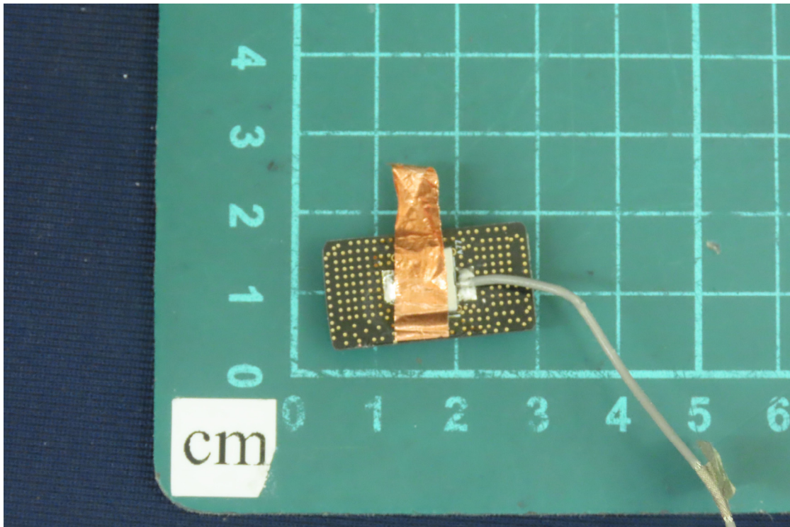
(65) EUT Photo
