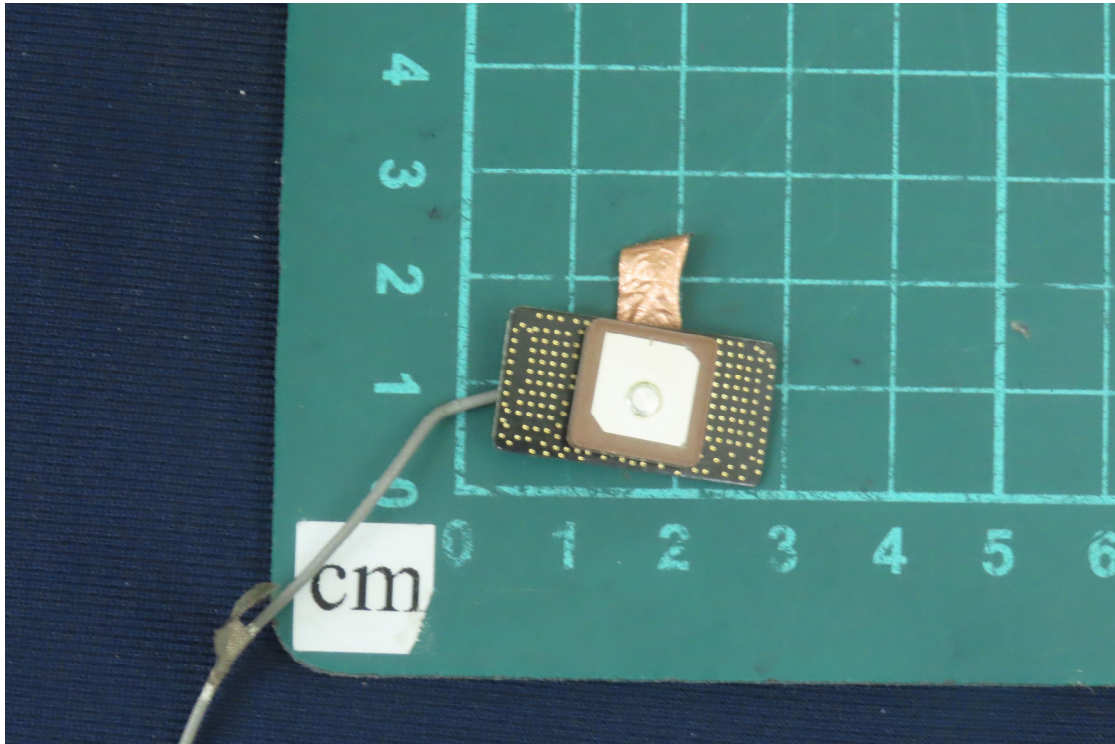
(64) EUT Photo
