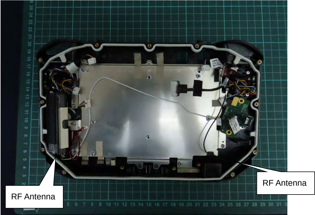
(46) EUT Photo
