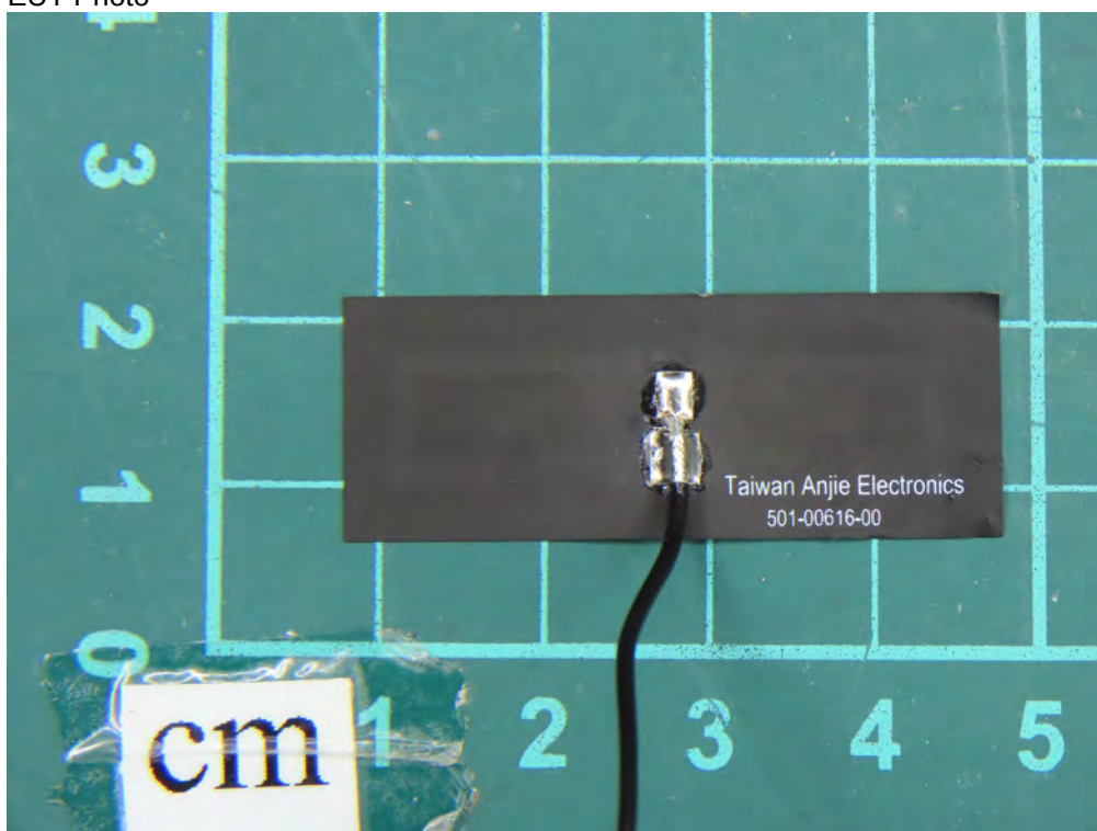
(50) EUT Photo
