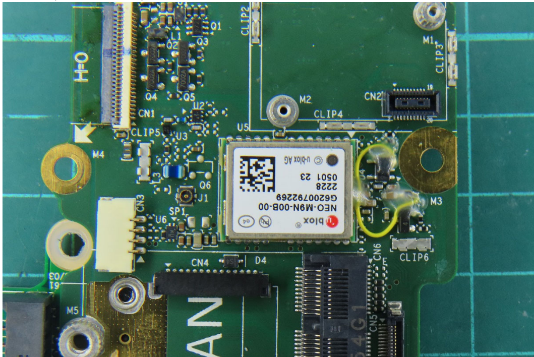
(23) EUT Photo (GPS module)
