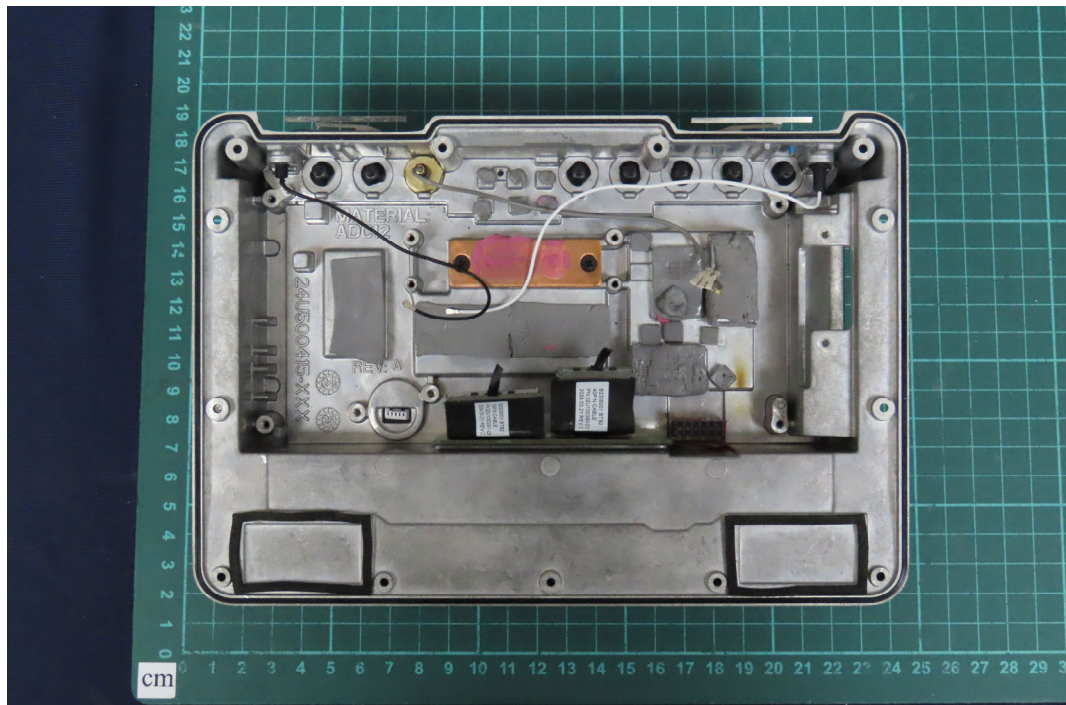
(46) EUT Photo
