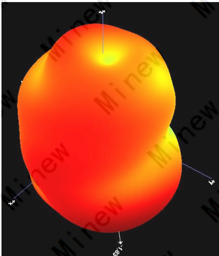
2402MHz
