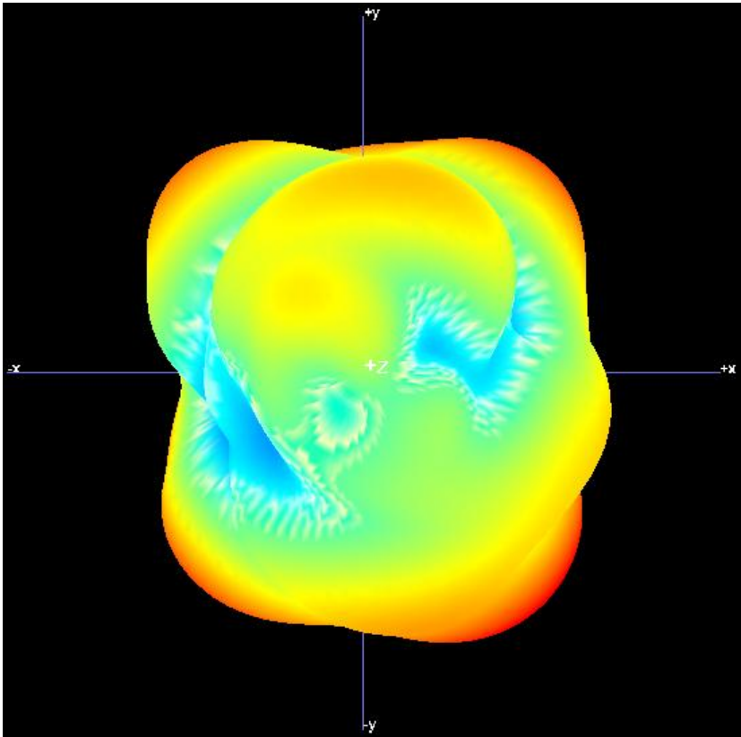
2440MHz
