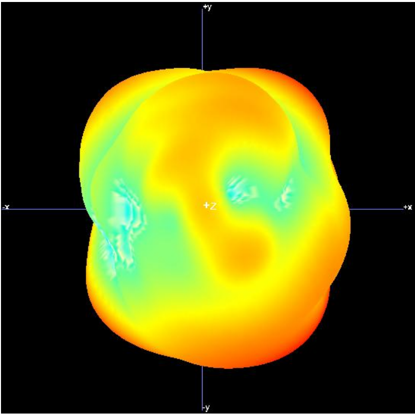
2402MHz
