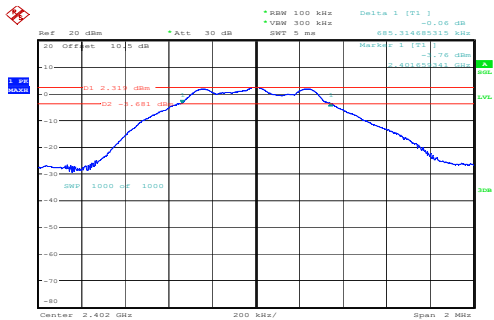
Low 0.685MHz
