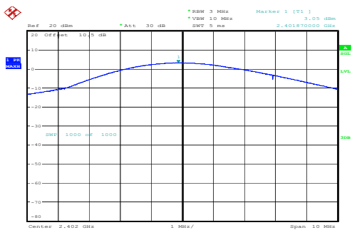
Low 3.05dBm
