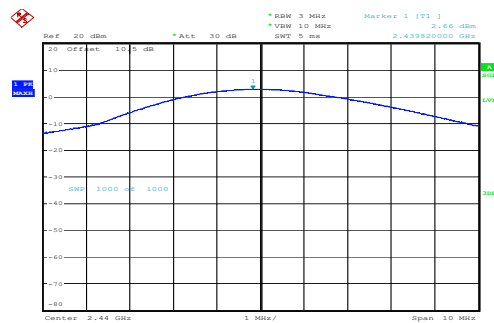
Middle 2.66dBm
