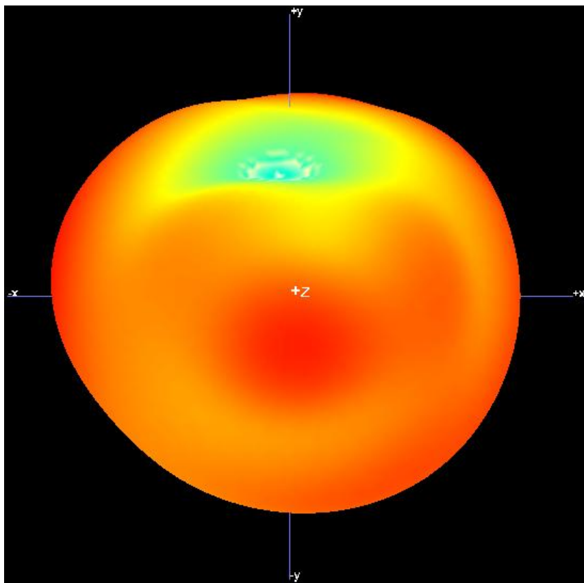
2480MHz
