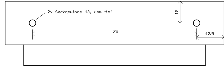
Außenansicht
