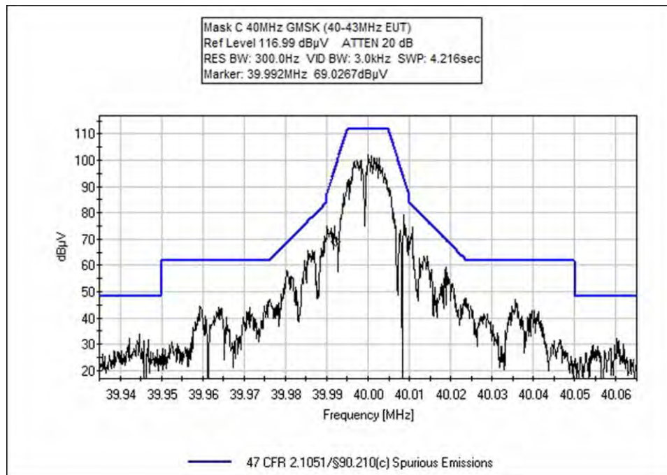
40MHz, GMSK
