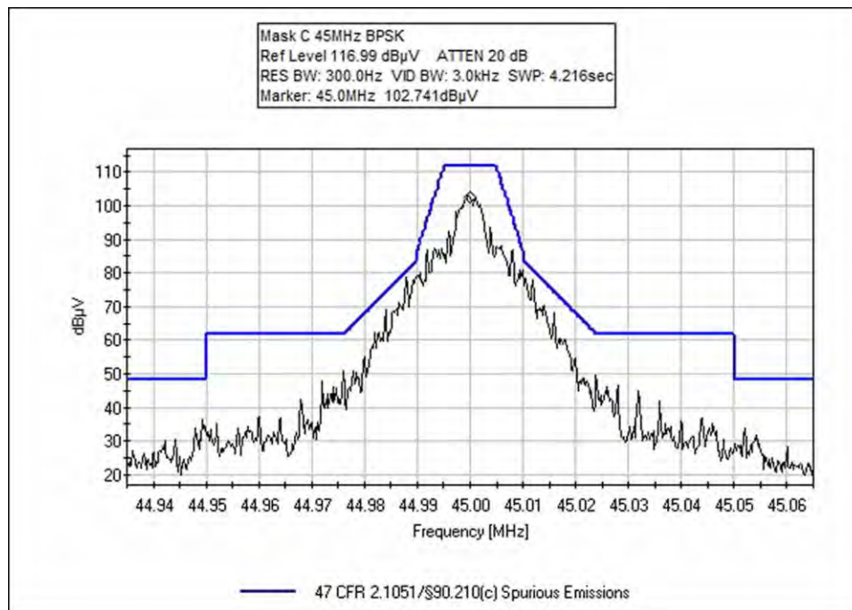
45MHz, BPSK
