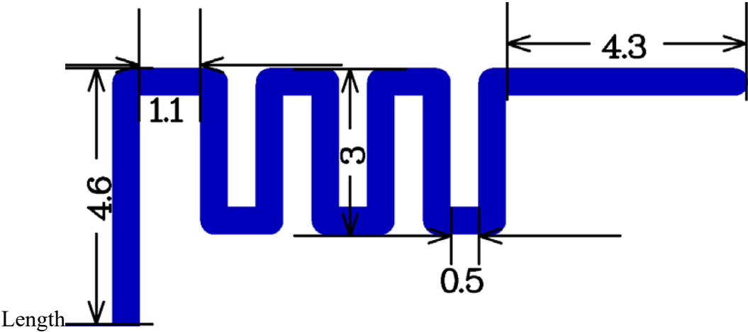
Antenna Photo & （单位： mm）
