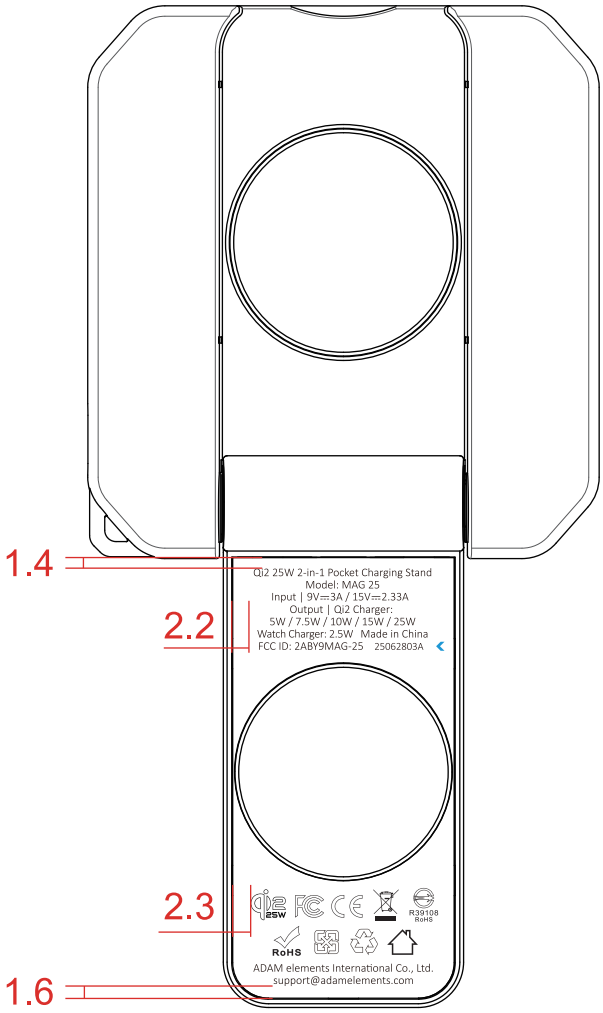
後視圖(支架轉至底)
