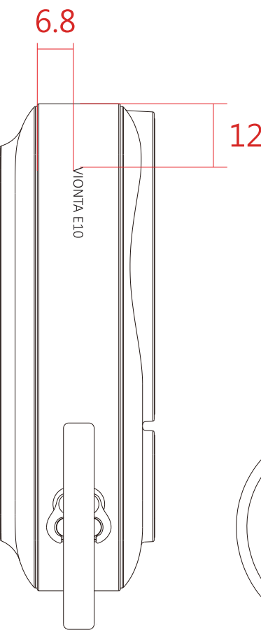
左視圖
