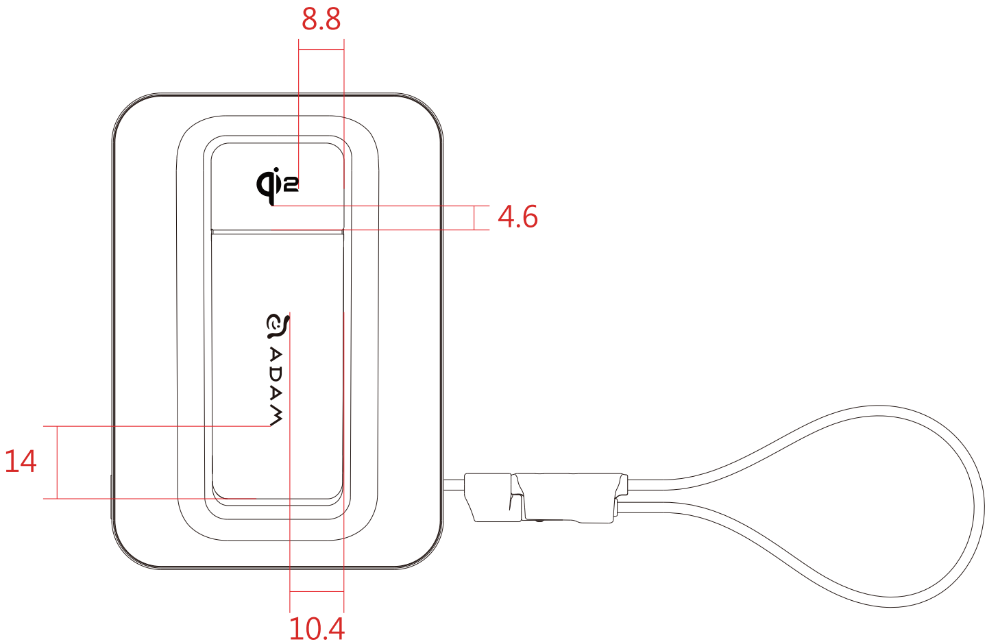
後視圖
