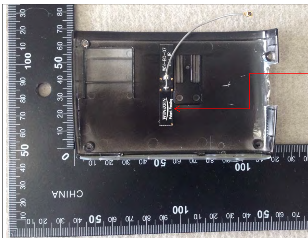
RF Module
