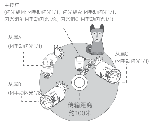
使用三个从属灯进行无线闪光拍摄
