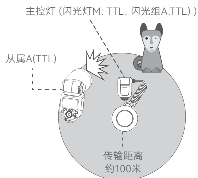
使用一个从属灯进行自动闪光拍摄
