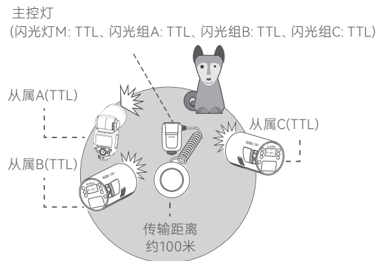
使用三个从属灯进行自动闪光拍摄
