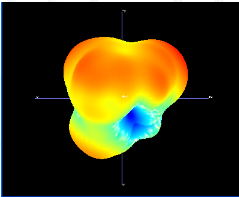
2450MHz
