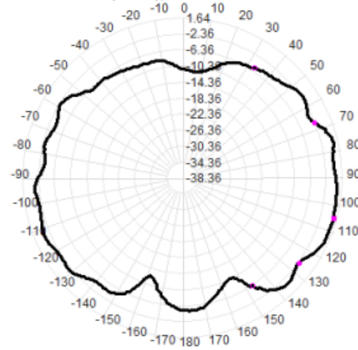
2441.0MHz Total(E2-YZ), Max= 0.53dBi
