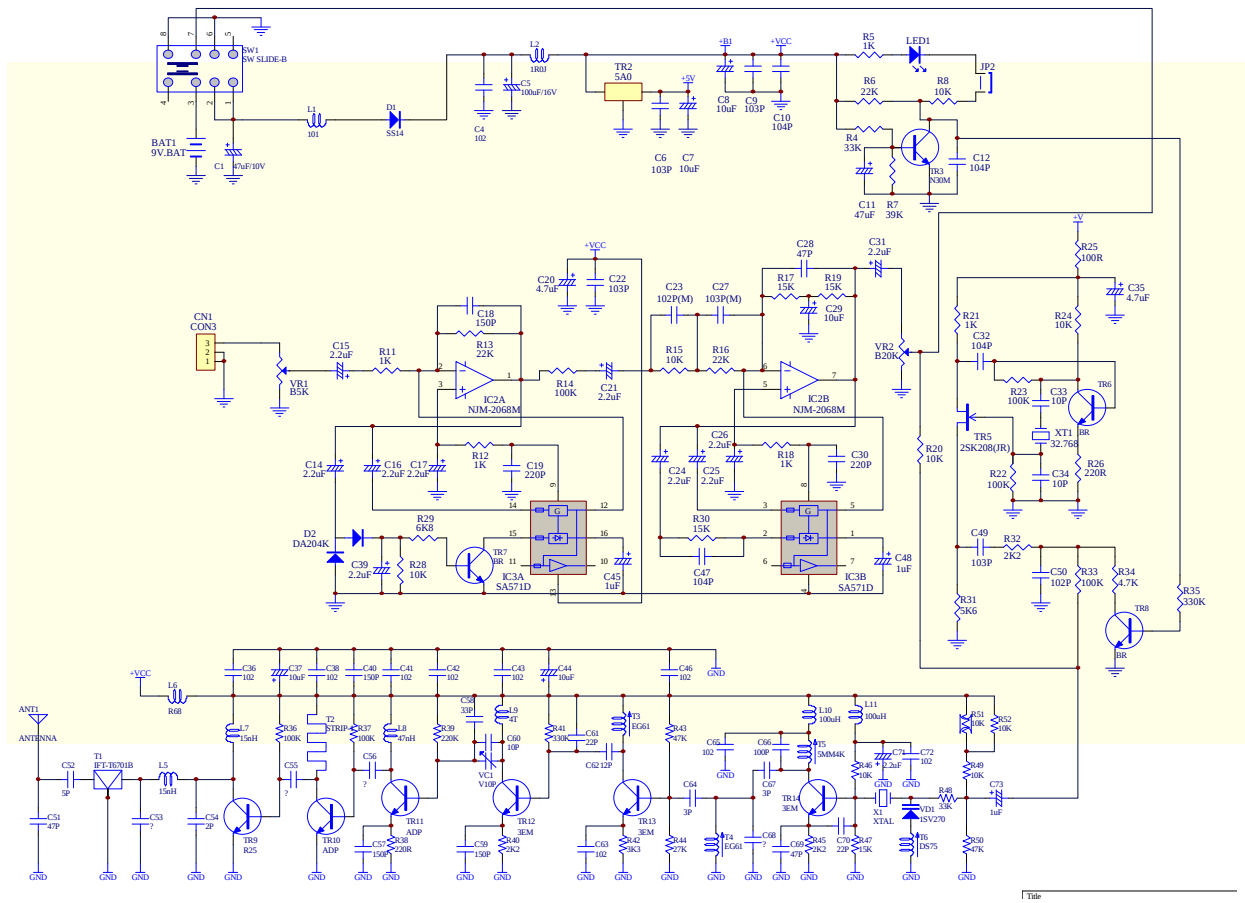
transmitter 原理图
