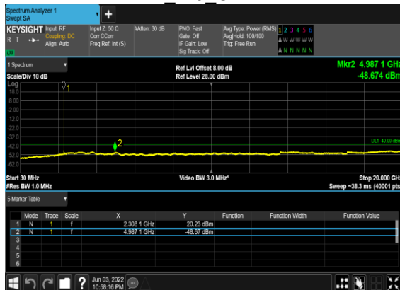
B5_N30(5M)_DFT-s-OFDM_BPSK_Edge_1RB_Left Mid CH
