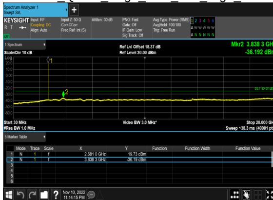
N41(10M)_CP- OFDM QPSK Edge 1RB Left High CH
