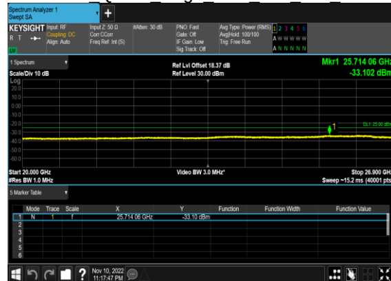
N41(50M)_CP- OFDM QPSK Edge 1RB Left Mid CH
