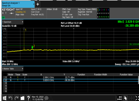
N41(10M)_CP- OFDM QPSK Edge 1RB Left Mid CH
