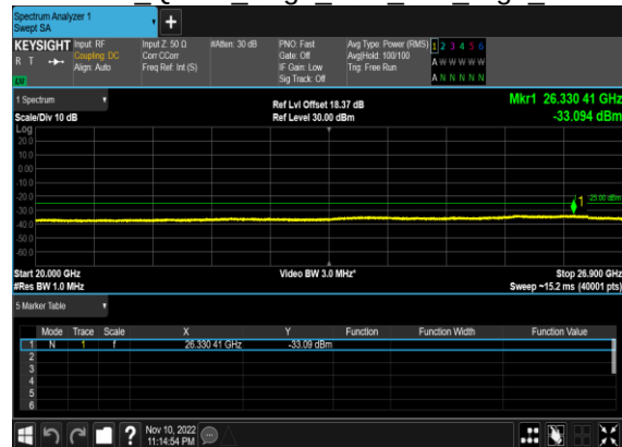
N41(10M)_CP- OFDM QPSK Edge 1RB Left High CH
