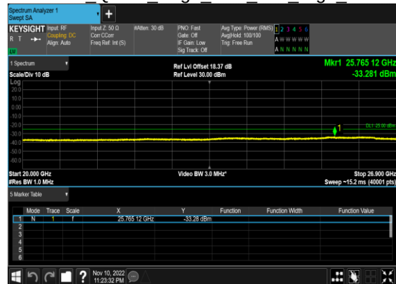
N41(100M)_CP- OFDM QPSK Edge 1RB Left High CH
