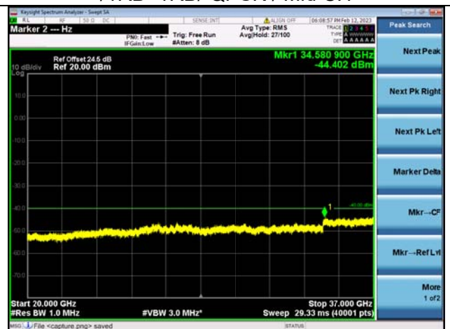
Band48C-20G-37G / 10MHz+20MHz /50RB+100RB/ QPSK / Mid CH
