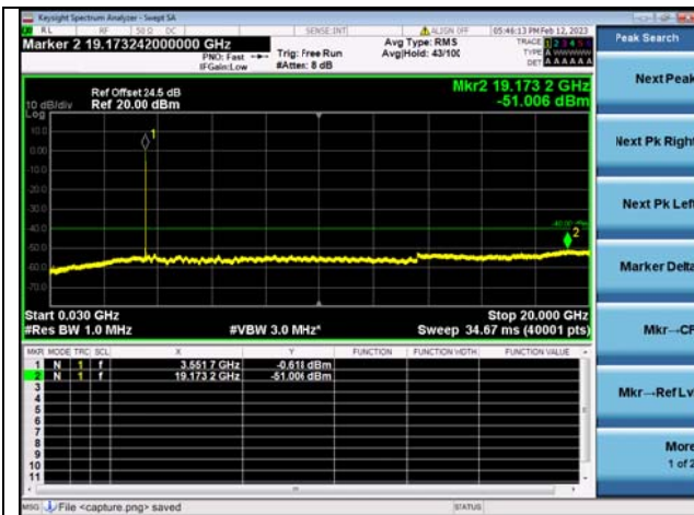
Band48C-30M-20G / 20MHz+10MHz /1RB+1RB/ QPSK / Low CH
