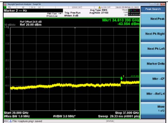
Band48C-20G-37G / 5MHz+20MHz / 1RB+1RB / QPSK / Mid CH
