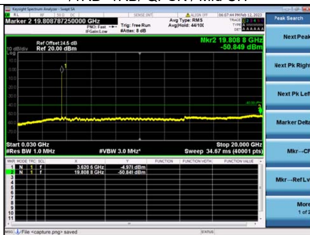
Band48C-30M-20G / 10MHz+20MHz /1RB+1RB/ QPSK / Mid CH
