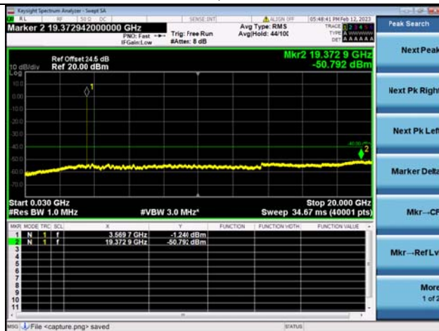
Band48C-30M-20G / 20MHz+10MHz /1RB+1RB/ QPSK / Low CH
