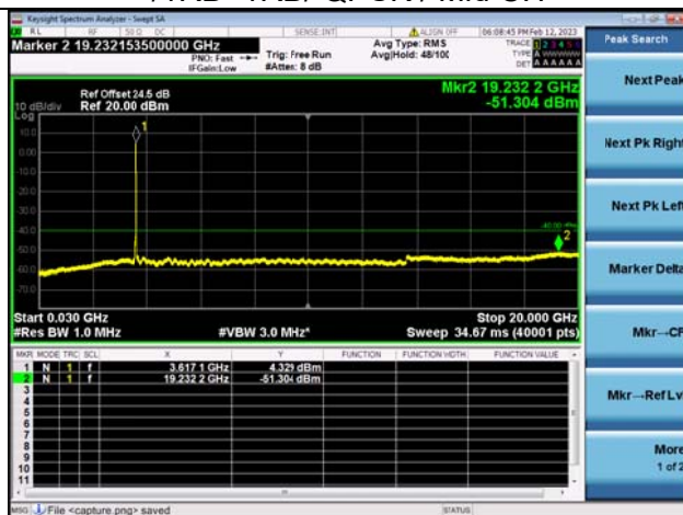
Band48C-30M-20G / 10MHz+20MHz /50RB+100RB/ QPSK / Mid CH
