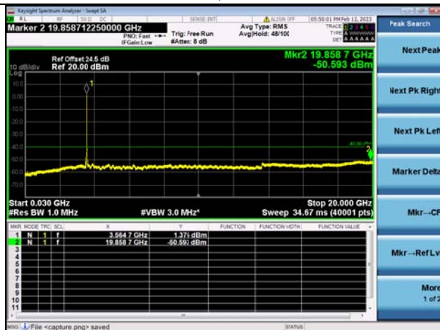
Band48C-30M-20G / 20MHz+10MHz /100RB+50RB/ QPSK / Low CH
