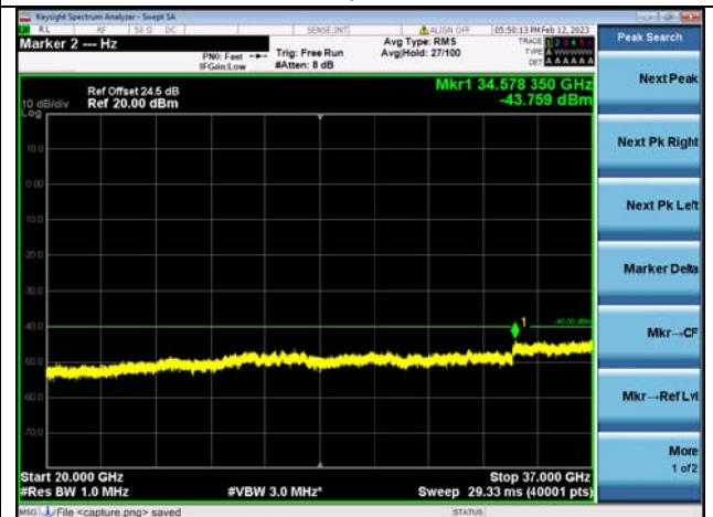
Band48C-20G-37G / 20MHz+10MHz /100RB+50RB/ QPSK / Low CH
