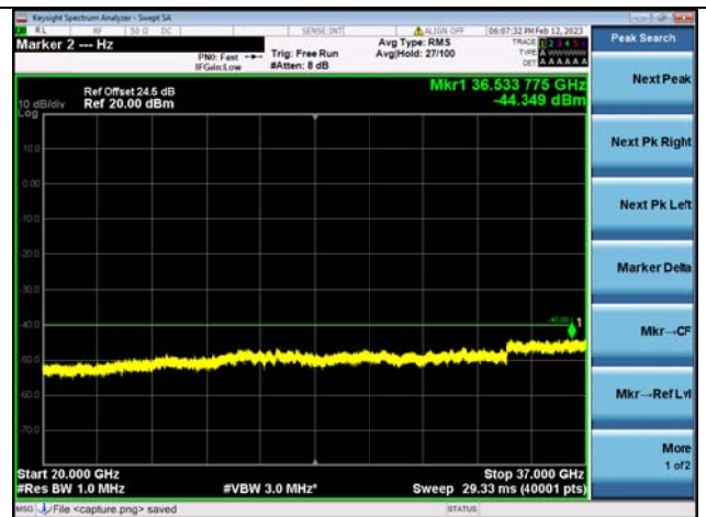
Band48C-20G-37G / 10MHz+20MHz /1RB+1RB/ QPSK / Mid CH
