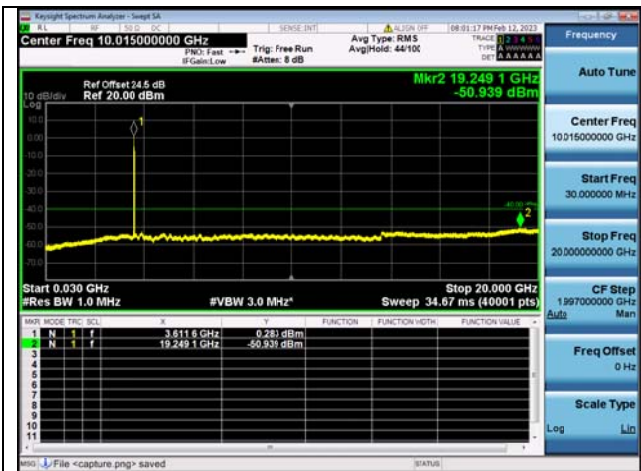
Band48C-30M-20G / 10MHz+20MHz /1RB+1RB/ QPSK / Mid CH
