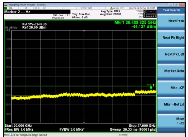
Band48C-20G-37G / 20MHz+5MHz / 1RB+1RB / QPSK / High CH
