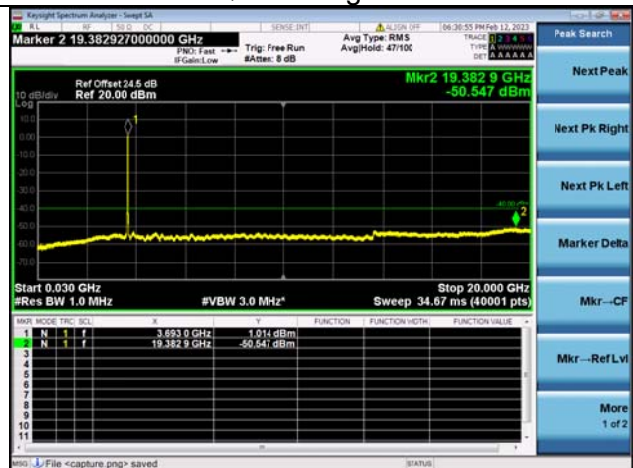
Band48C-30M-20G / 20MHz+5MHz / 100RB+25RB / QPSK / High CH
