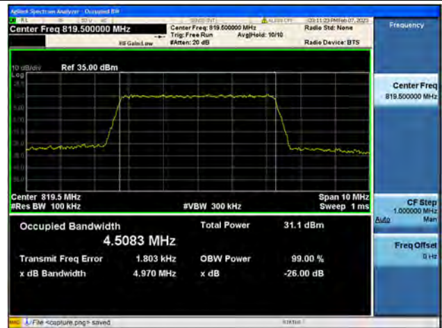
Band18Part90 / 5MHz / QPSK/ Mid CH
