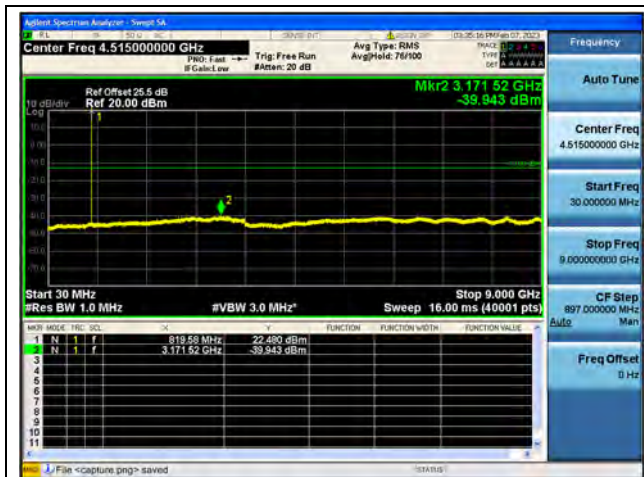
Band18Part90 / 5MHz / High CH / QPSK
