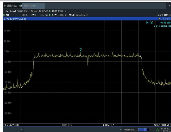
11BE40MIMO_Ant2_2422_0~Reference
