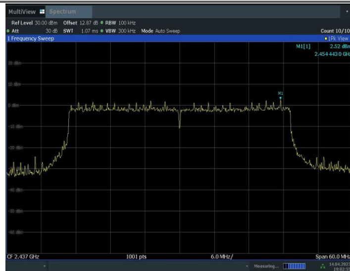
11BE40MIMO_Ant2_2437_0~Reference
