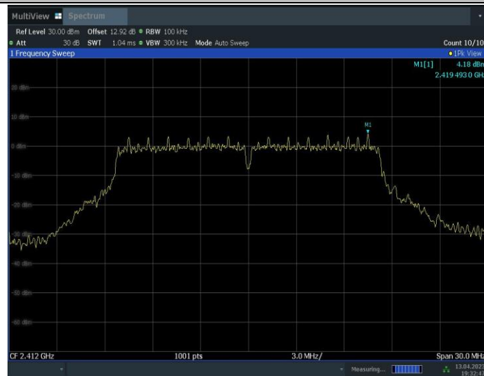
11G-CDD_Ant2_2412_0-Reference
