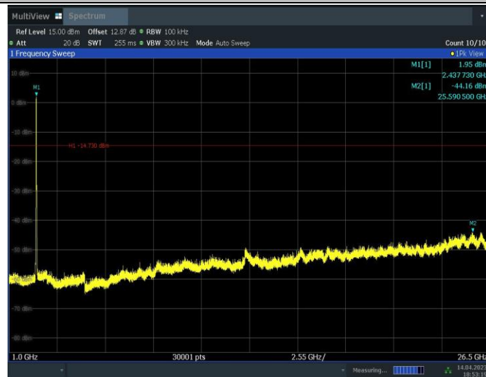
11BE20MIMO_Ant2_2437_1000~26500
