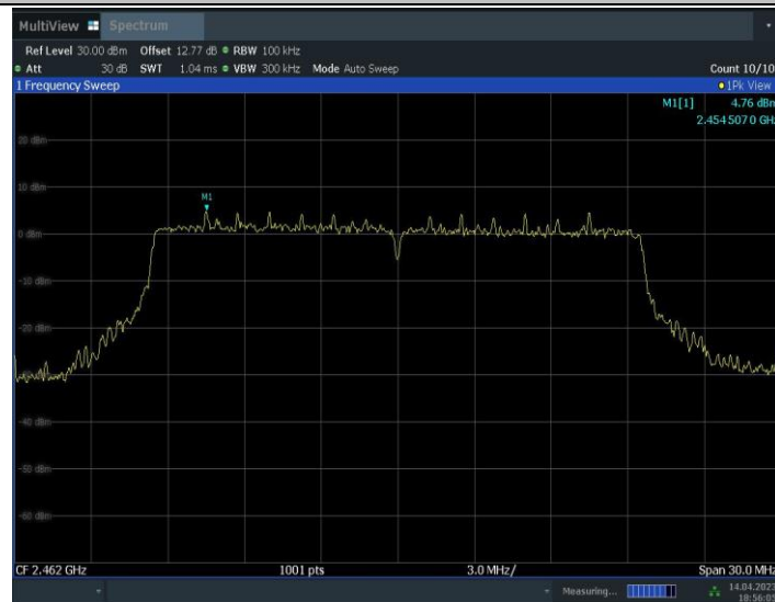
11BE20MIMO_Ant2_2462_0~Reference
