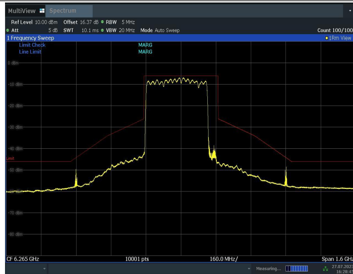
11BE320MIMO_Ant2_6265_996+996+996_1
