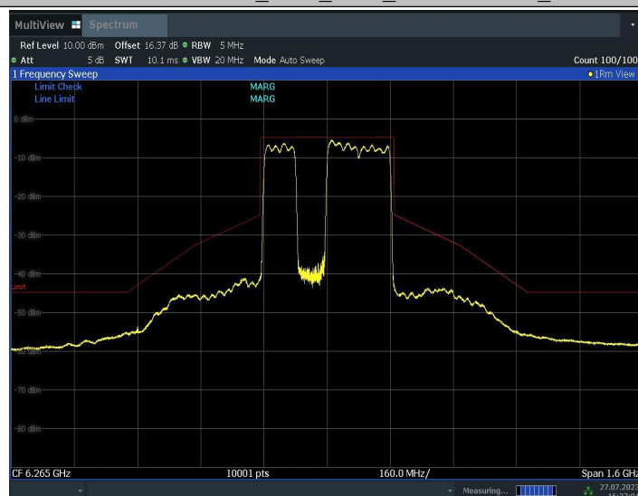
11BE320MIMO_Ant2_6265_996+996+996_2
