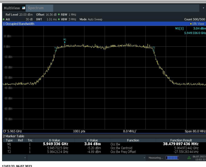
11BE40MIMO_Ant1_5965
