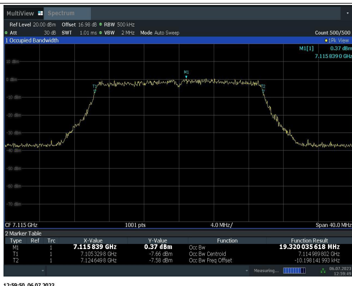
11BE20MIMO_Ant2_7115
